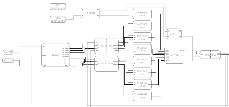
Figura 2.2 — Schema conexiunilor dintre placă, izolatoare, convertor și servomotoare.
