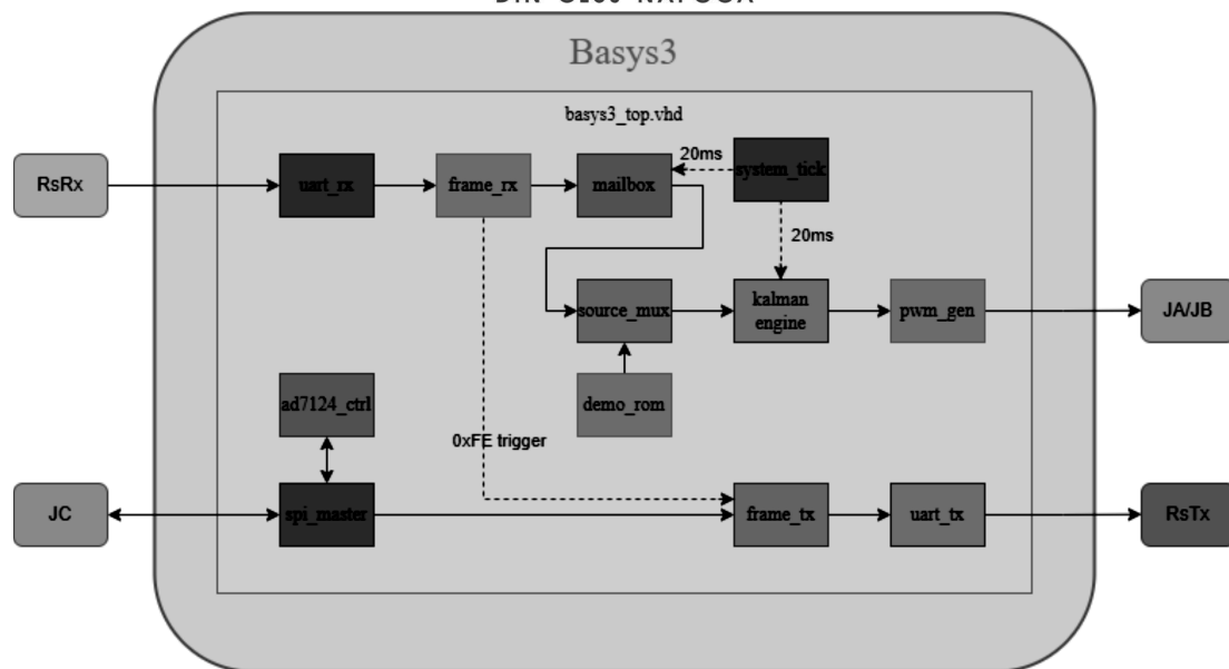
Figura 2.1 — Arhitectura modulelor VHDL implementate pe placa Basys3.
