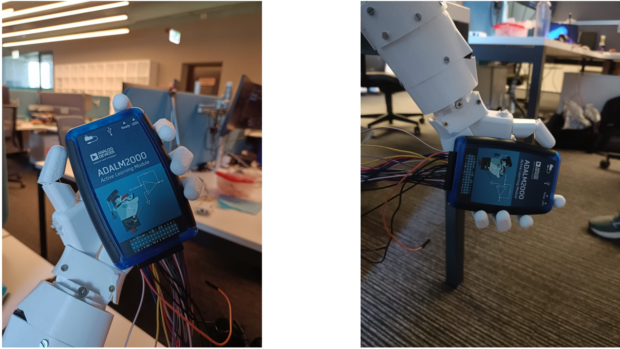
Figura 6.2: Mâna robotică prinzând un modul electronic, văzută din două unghiuri.
