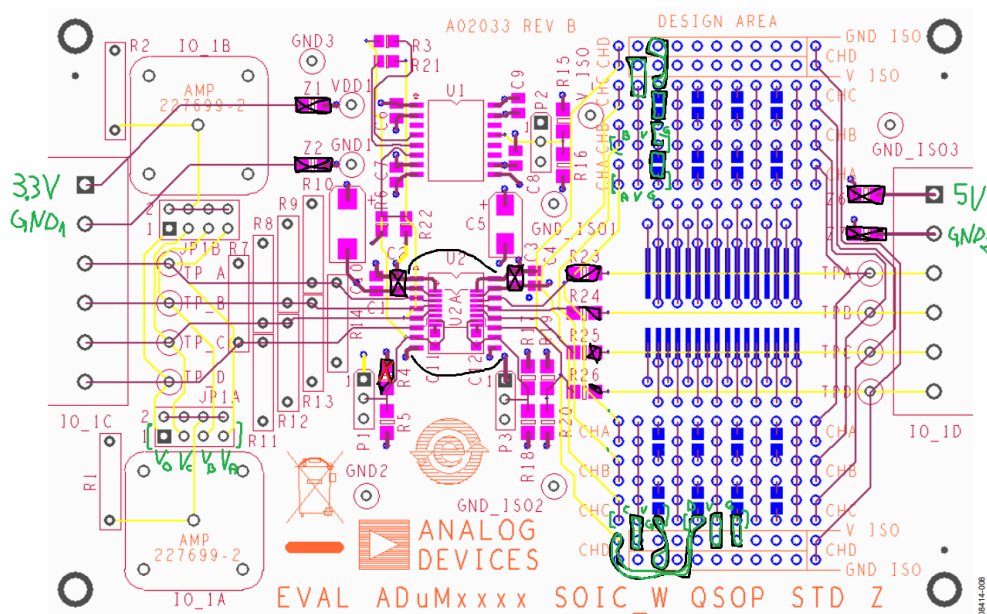
Figura 1.10: Amplasarea componentelor pe zona de prototipare a plăcii de evaluare ADuM1400. Cu verde sunt marcate canalele pentru pinii servomotoarelor.
