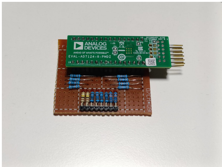
Figura 1.7: Plăcuța cu divizoarele rezistive de atenuare și convertorul AD7124-8.
