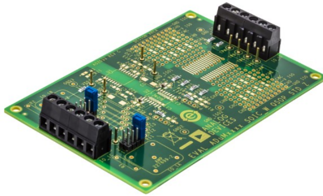
Figura 4.9: Placa de evaluare pe care se montează izolatorul ADuM1400 [16], cu conexiunile aduse la borne accesibile pentru integrarea în montaj.
