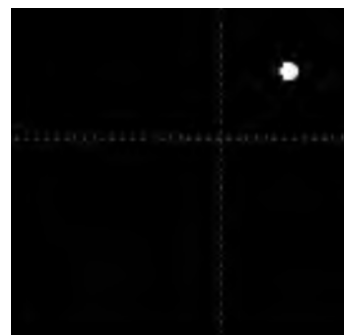
图 12. 源星体偏离对称轴且完全超出临界源平面时的成像示意 图片来源：陈品健, 刘海程, 李向华: 基于坐标变换的引力透镜模拟. 大学物理, 2023, 42, 54[2]
