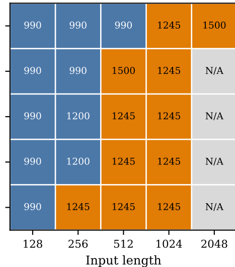
(b) P99 TTFT \leq 5000 ms
