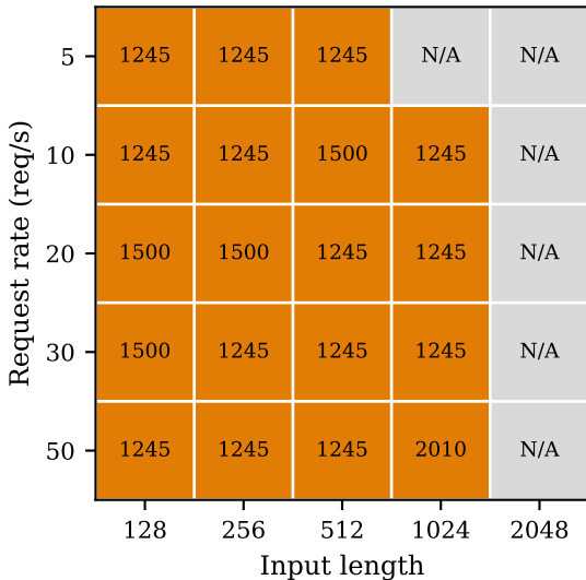
(a) P99 TTFT \leq 100 ms
