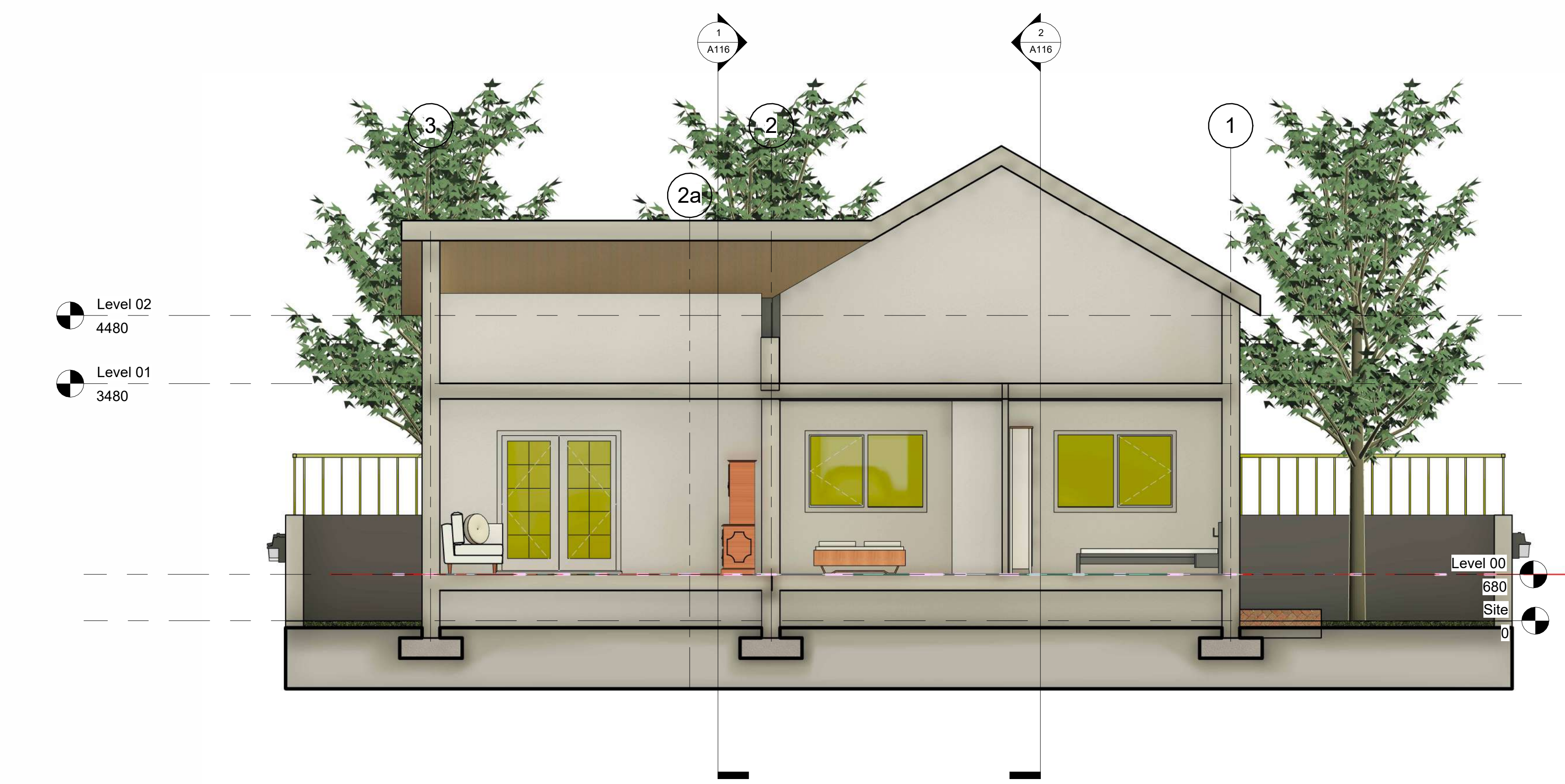
3 Section 5 1 : 50
