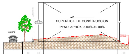
VISTA LATERAL ALTURA MAXIMA DE 8.50 MTS. NO PUEDE EXCEDER DOS NIVELES COMO MAXIMO
