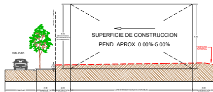
VISTA LATERAL ALTURA MAXIMA DE 8.50 MTS. NO PUEDE EXCEDER DOS NIVELES COMO MAXIMO LA PENDIENTE PUEDE SER POSITIVA O NEGATIVA
