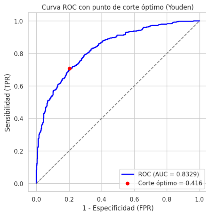
Figura 4. Curva ROC con el punto de corte óptimo de Youden
