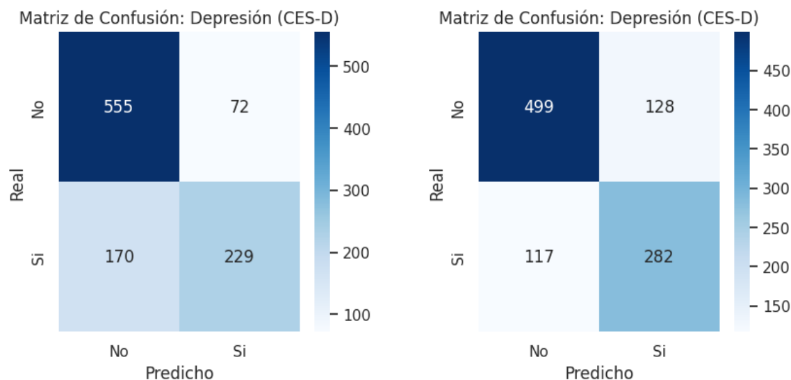
Figura 9. Matrices de confusión con el umbral de 0.5 (izquierda) y con el umbral de 0.4165 (derecha)
