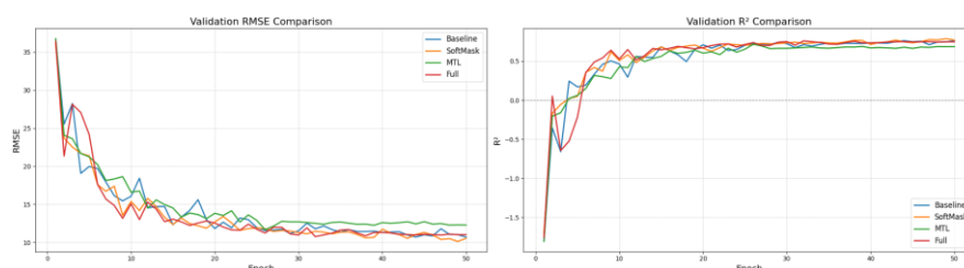
<Efficient-B0 四模型之RMSE及R²趨勢圖>
