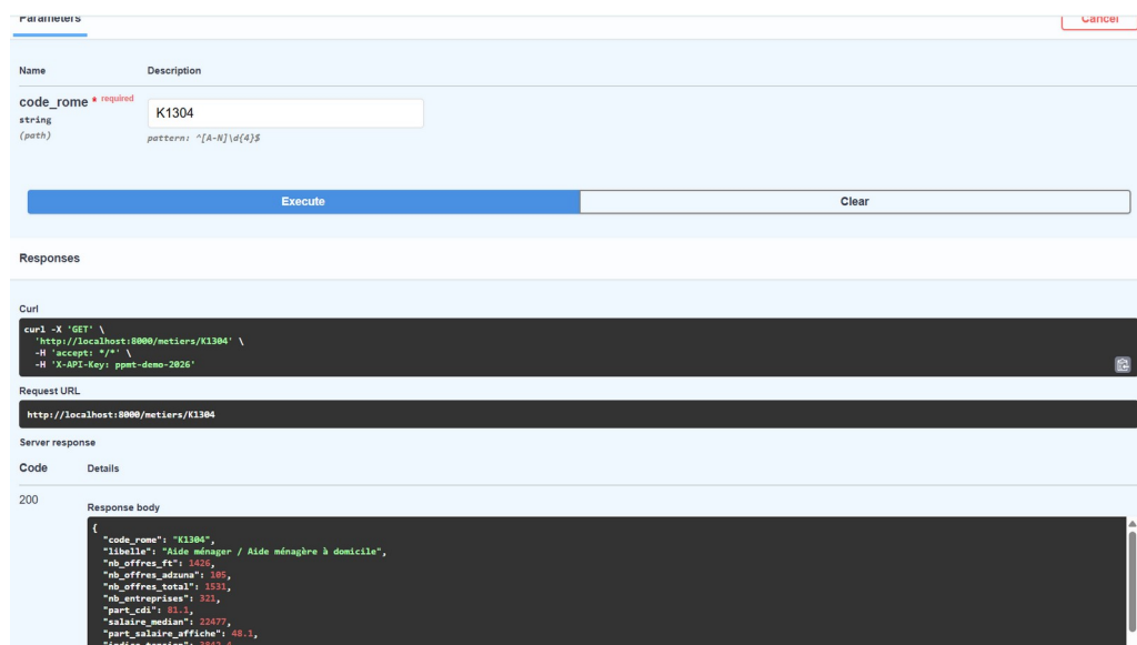
Figure 7 — Même appel depuis Swagger (« Try it out »)
