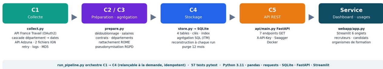
Figure 1 — Chaîne de traitement PPMT, des sources au service
