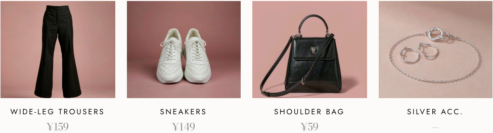
Fig. 04 — Match output.
