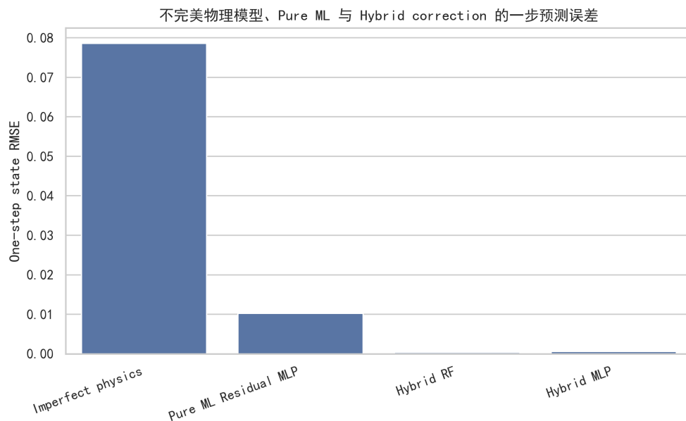
图 7: 不完美物理模型、Pure ML 与 Hybrid correction 的一步状态 RMSE 对比。Hybrid RF 和 Hybrid MLP 显著降低了由 \rho = 26 参数偏差引入的一步误差。
