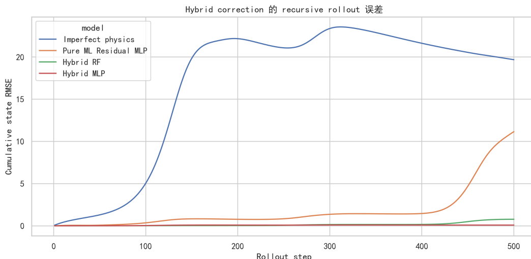
图 8: Hybrid correction 在递归多步推演中的累计状态 RMSE。Hybrid RF 和 Hybrid MLP 在当前 \rho = 26 参数偏差设定下保持更低误差，但该结论不应外推到所有物理模型错误。
