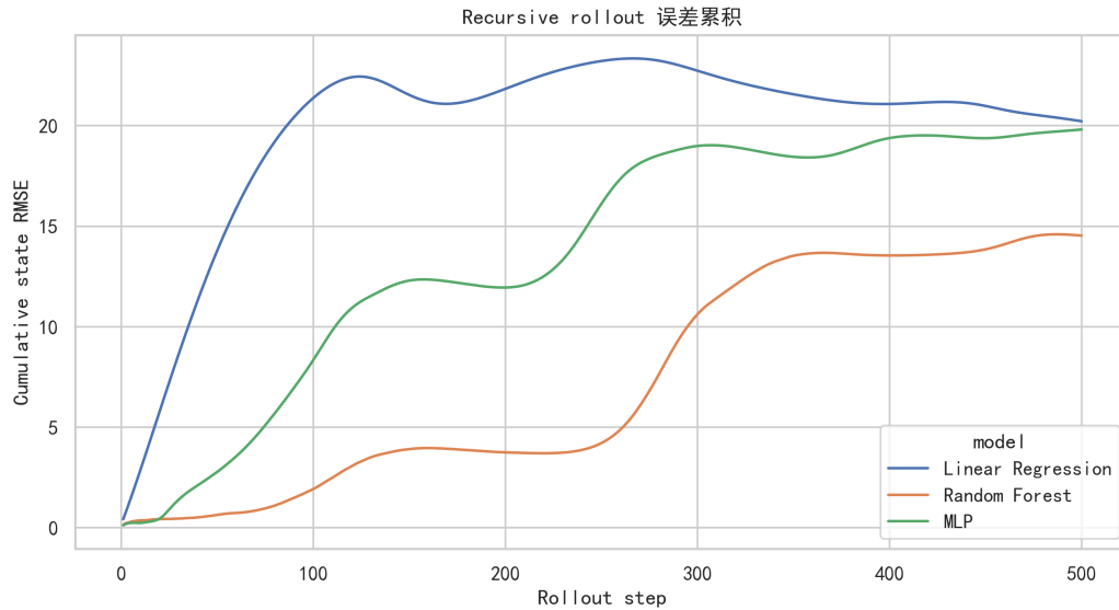
图 5: 递归多步推演中的误差累积曲线。模型自身误差会被反复输入下一步，因此短期一步误差会逐渐转化为长期轨迹偏离。
