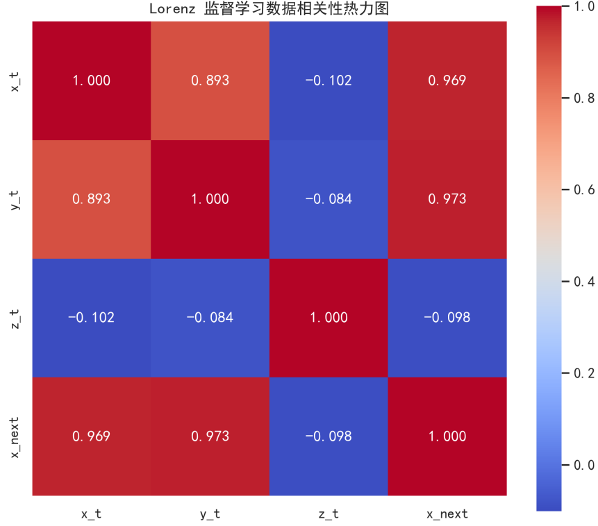
图 2: Lorenz 状态变量相关性热力图。该图用于展示不同特征之间的统计关系，是本文数据探索性分析的一部分。
