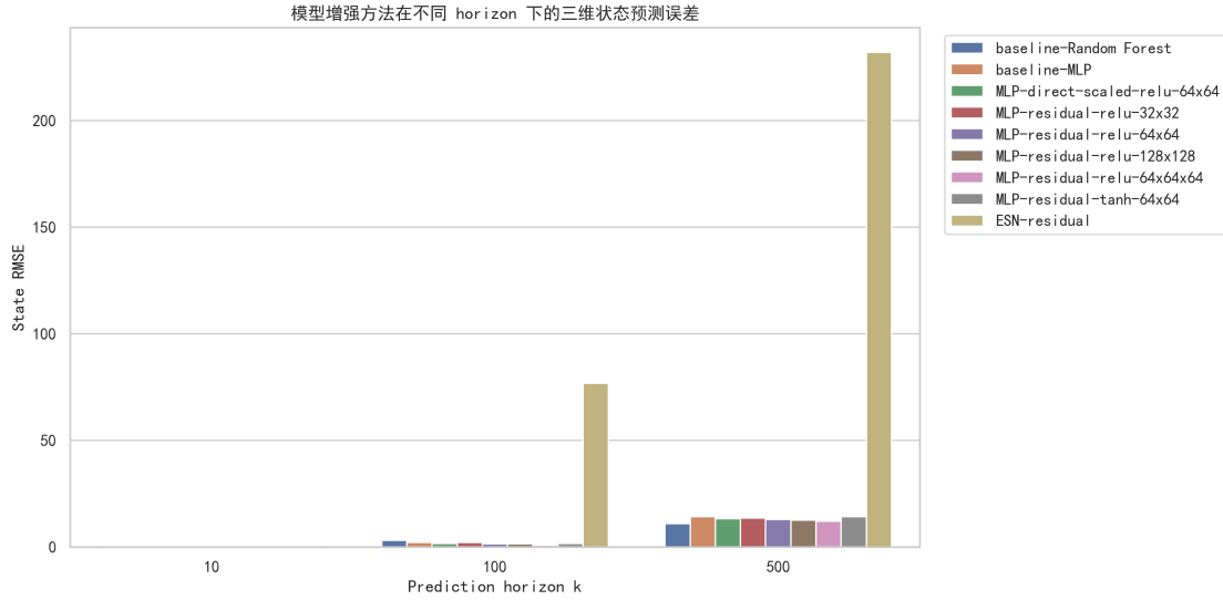
图 6: Residual MLP 与 Direct MLP 在不同 horizon 下的对比。残差学习在短中期明显降低误差，但较长 horizon 下仍受到混沌误差放大的限制。
