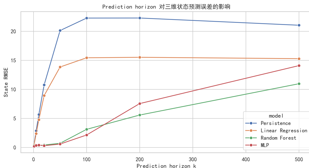
图 4: 不同 prediction horizon 下的状态 RMSE。随着 horizon 增大，各模型误差明显上升，说明普通监督学习模型的预测能力存在时间尺度边界。
