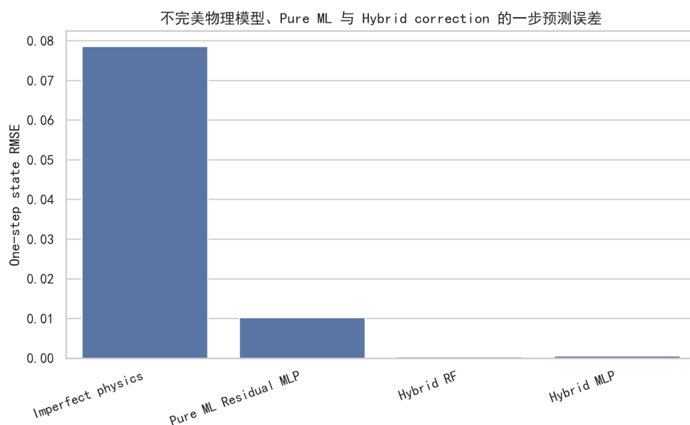
图 12: 不完美物理模型、Pure ML 与 Hybrid correction 的一步状态 RMSE 对比
