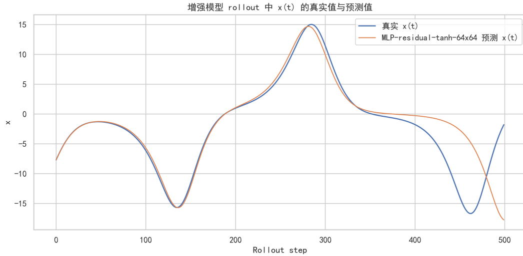
图 9: 增强模型递归多步预测中 x(t) 的真实值与预测值对比
