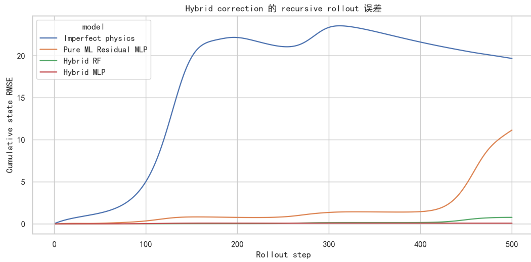
图 13: Hybrid correction 在递归多步预测中的累计状态 RMSE
