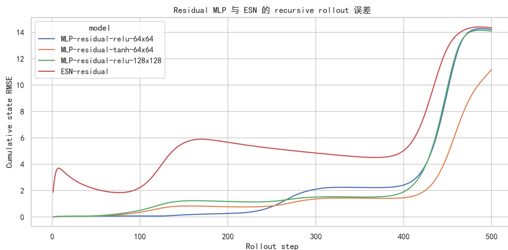
图 8: 增强模型递归多步预测误差曲线
