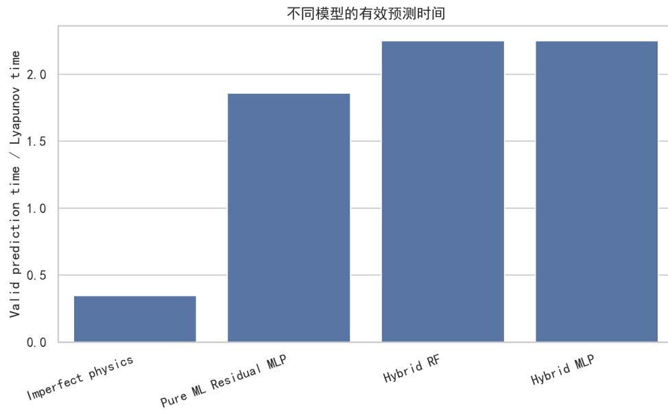
图 14: 不同模型的有效预测时间（以 Lyapunov time 归一化）
