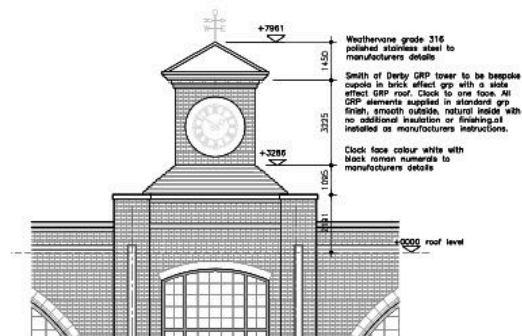
ELEVATION A scale:1:100
