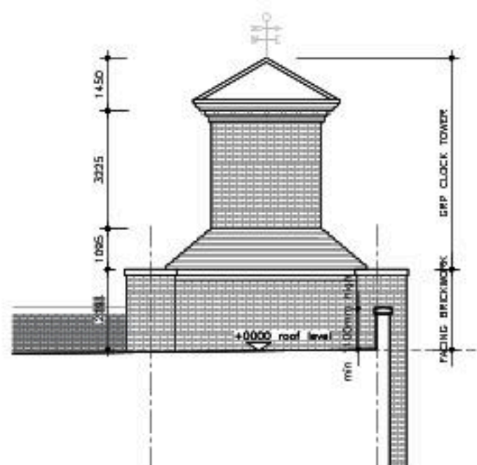
ELEVATION B
