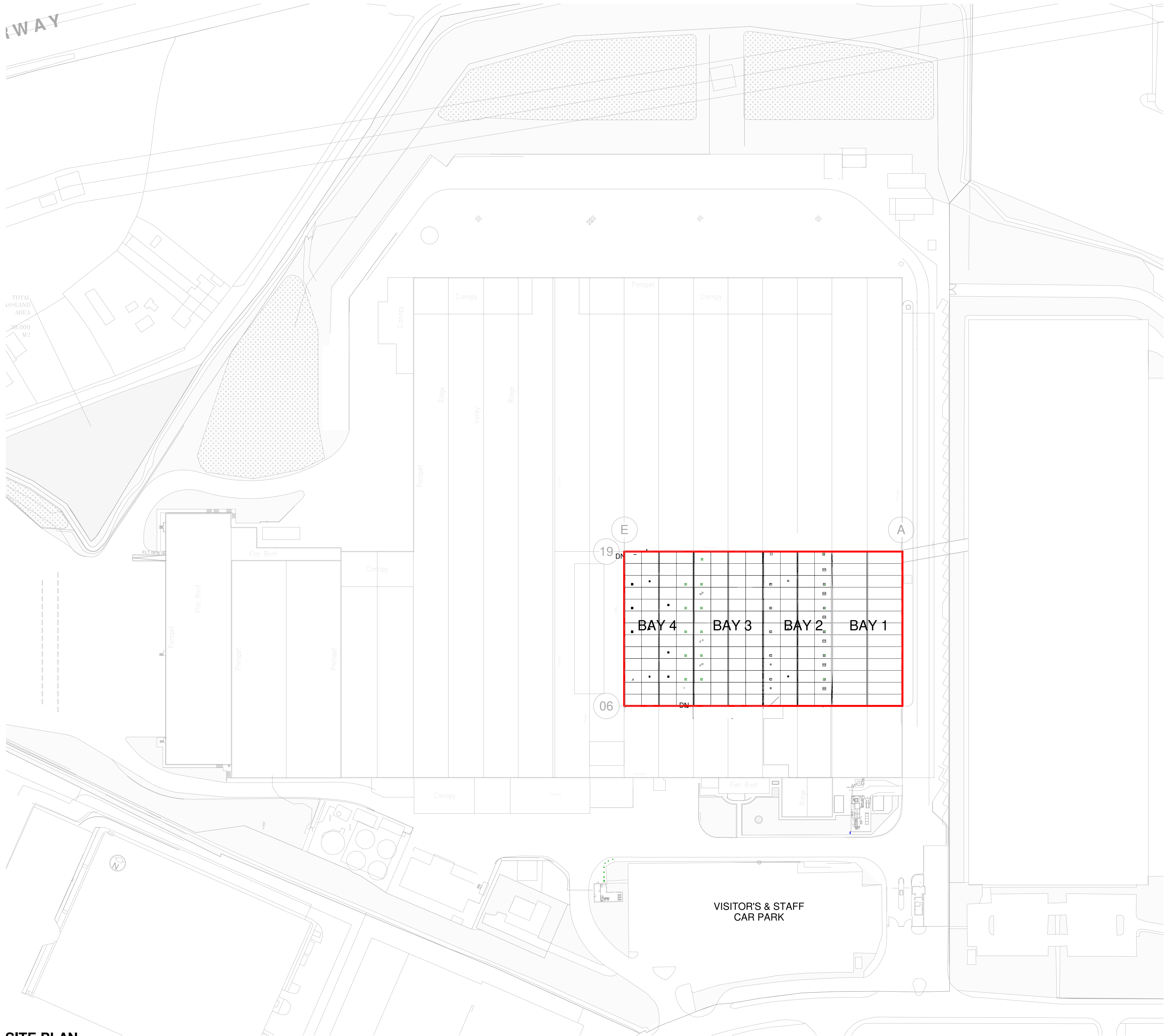
SITE PLAN 1 : 1000
