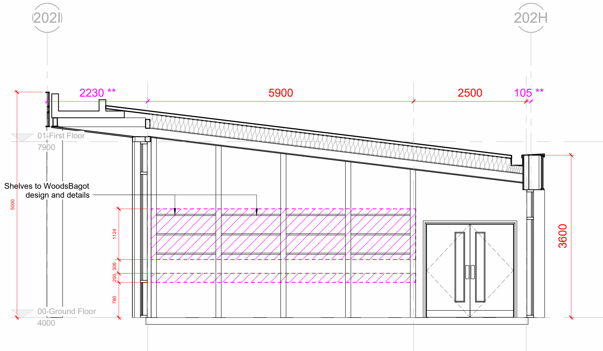
ELEVATION A 1 : 50
