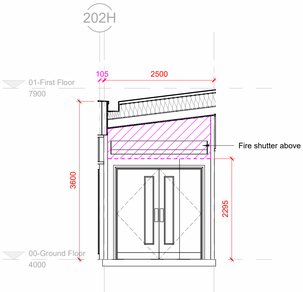
ELEVATION B 1 : 50
