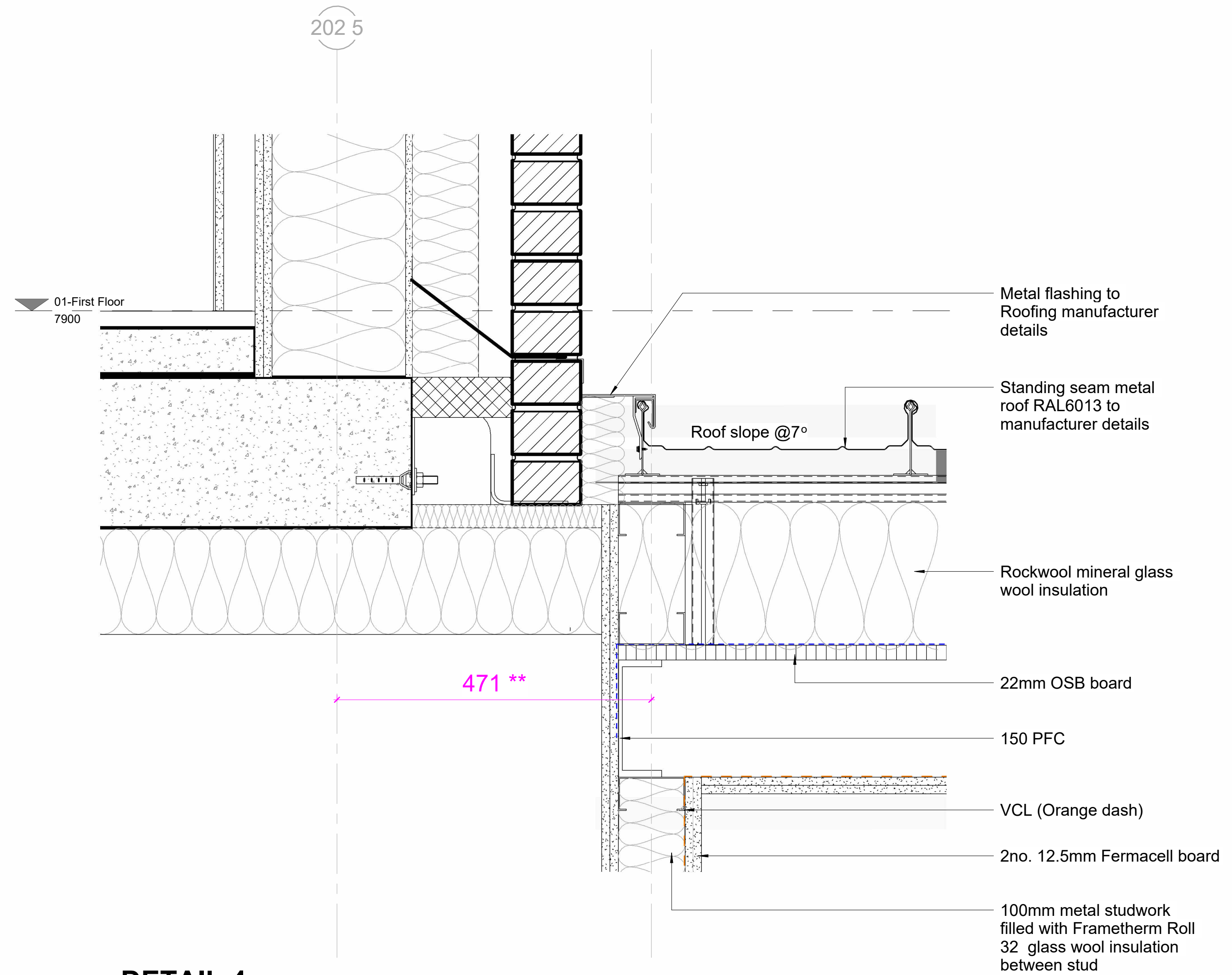
DETAIL 4 1 : 5
