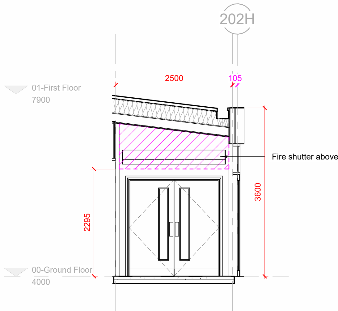
ELEVATION C 1 : 50
