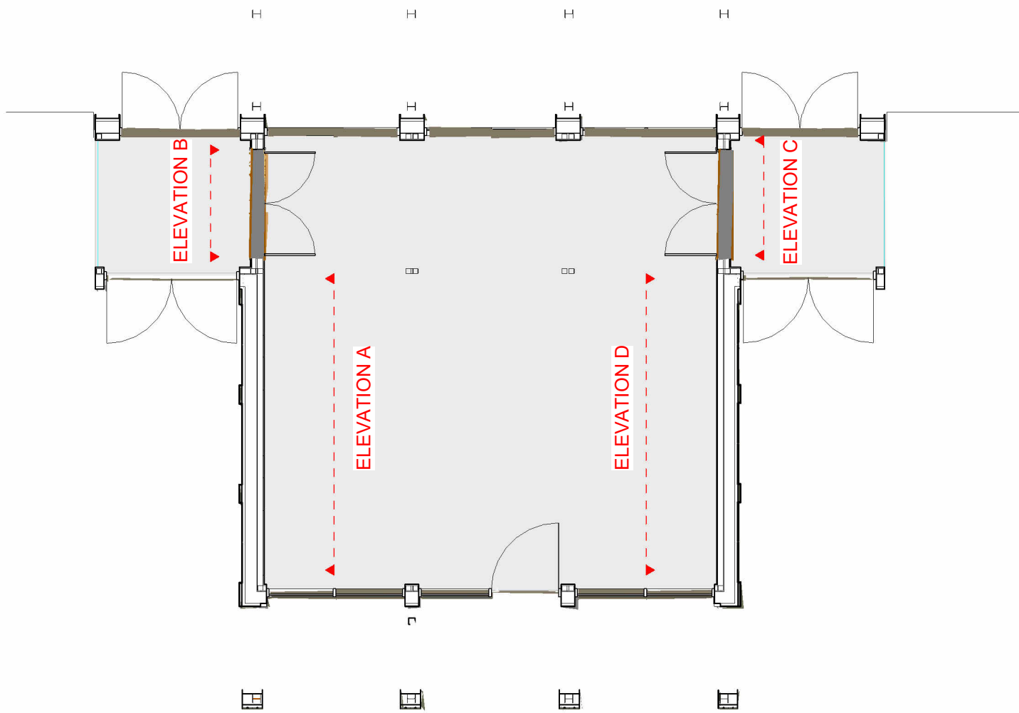
KEY PLAN 1 : 100
