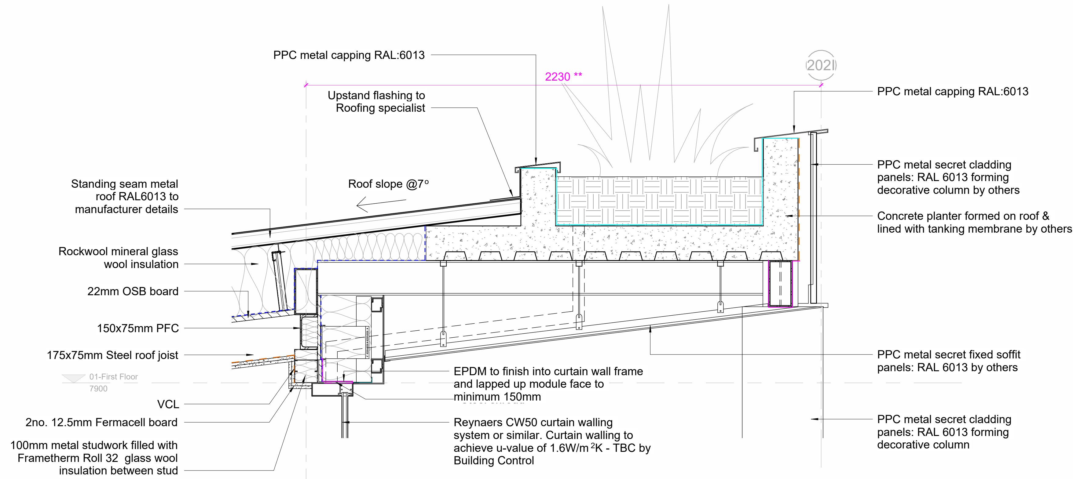
DETAIL 6 1 : 10
