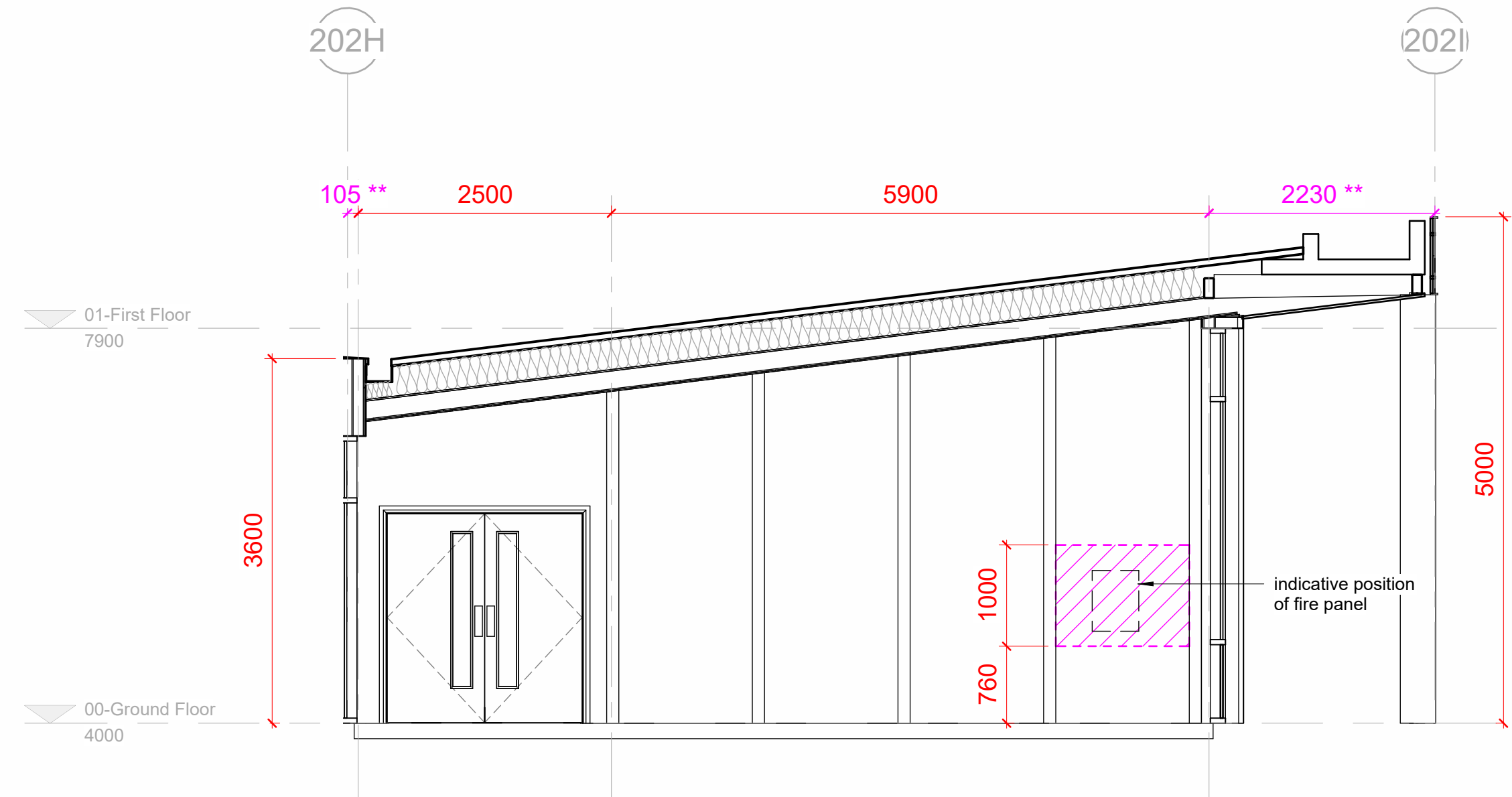
ELEVATION D 1 : 50
