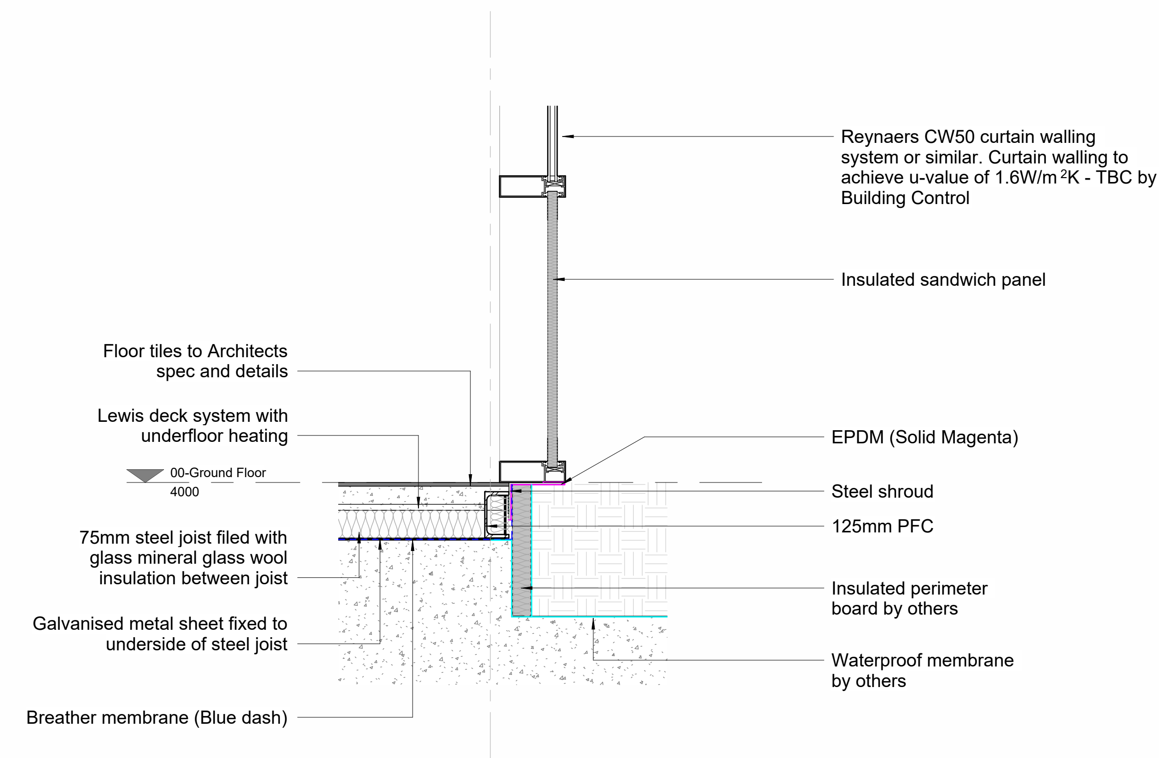
DETAIL 5 1 : 10
