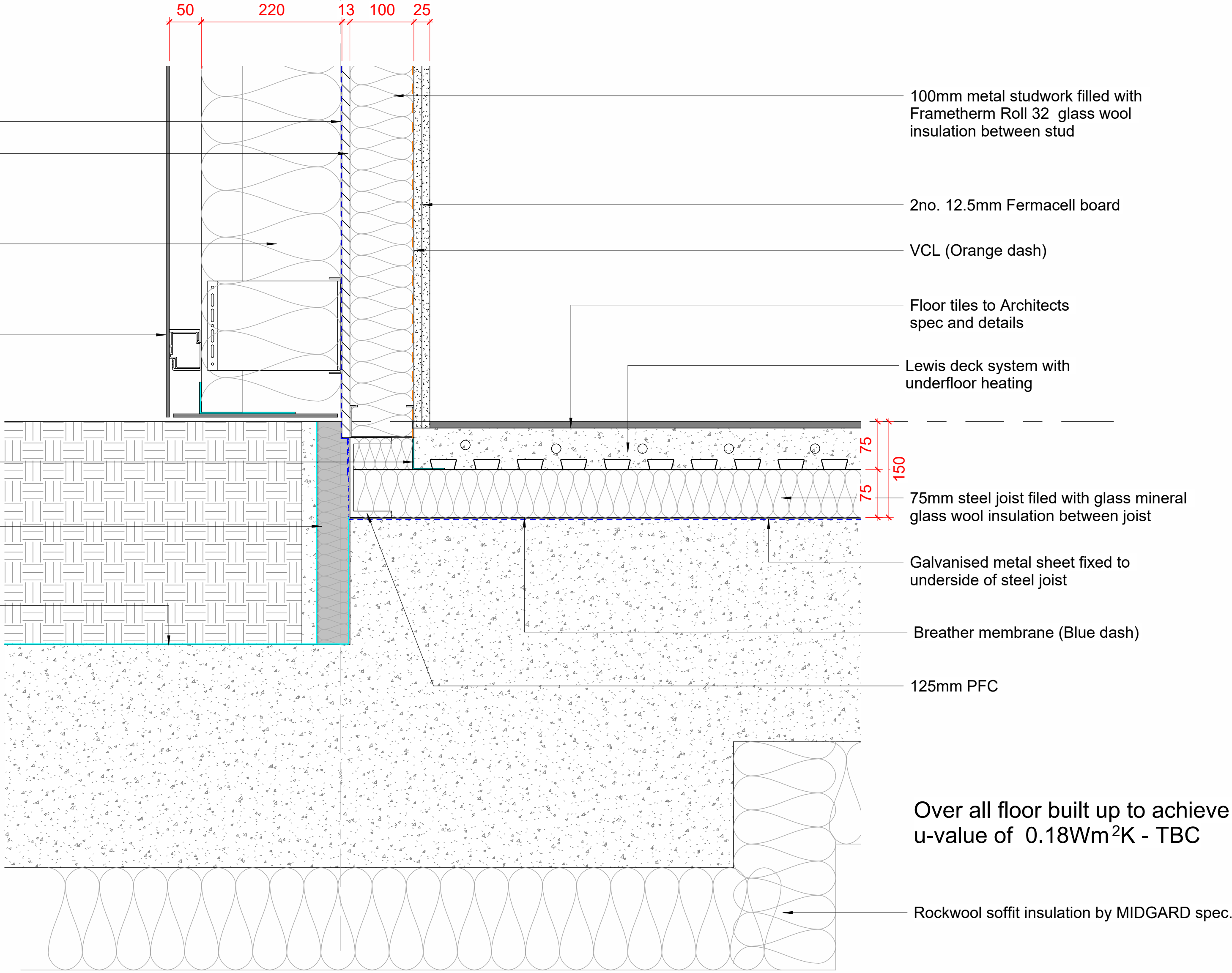
DETAIL 1 1 : 5
