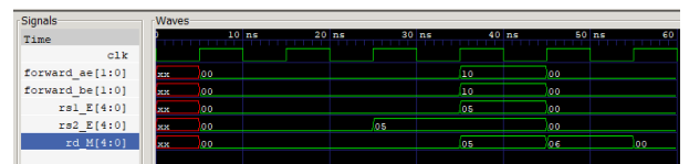
Fig. 2: mem - ex data hazard
