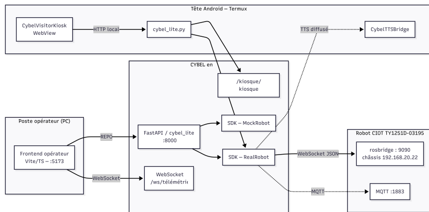
FIGURE 18 — Diagramme de composants (diagramme/diagramme_composant.png)
