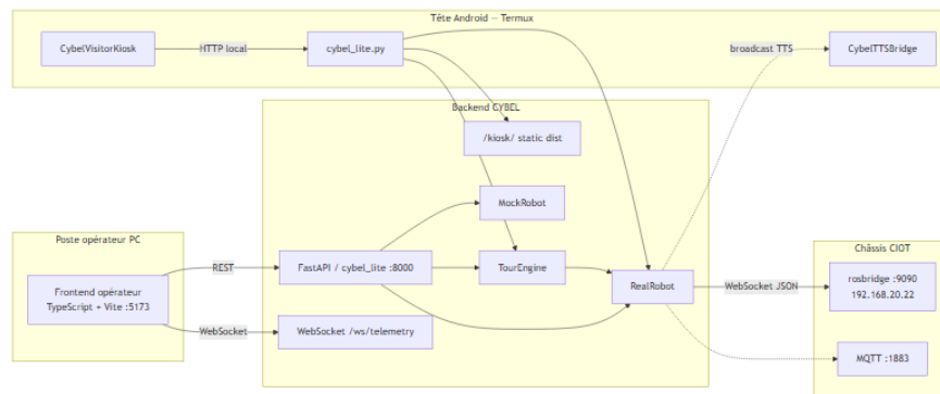
FIGURE 21 — Diagramme de composants (diagramme/diagramme_composant.png)
