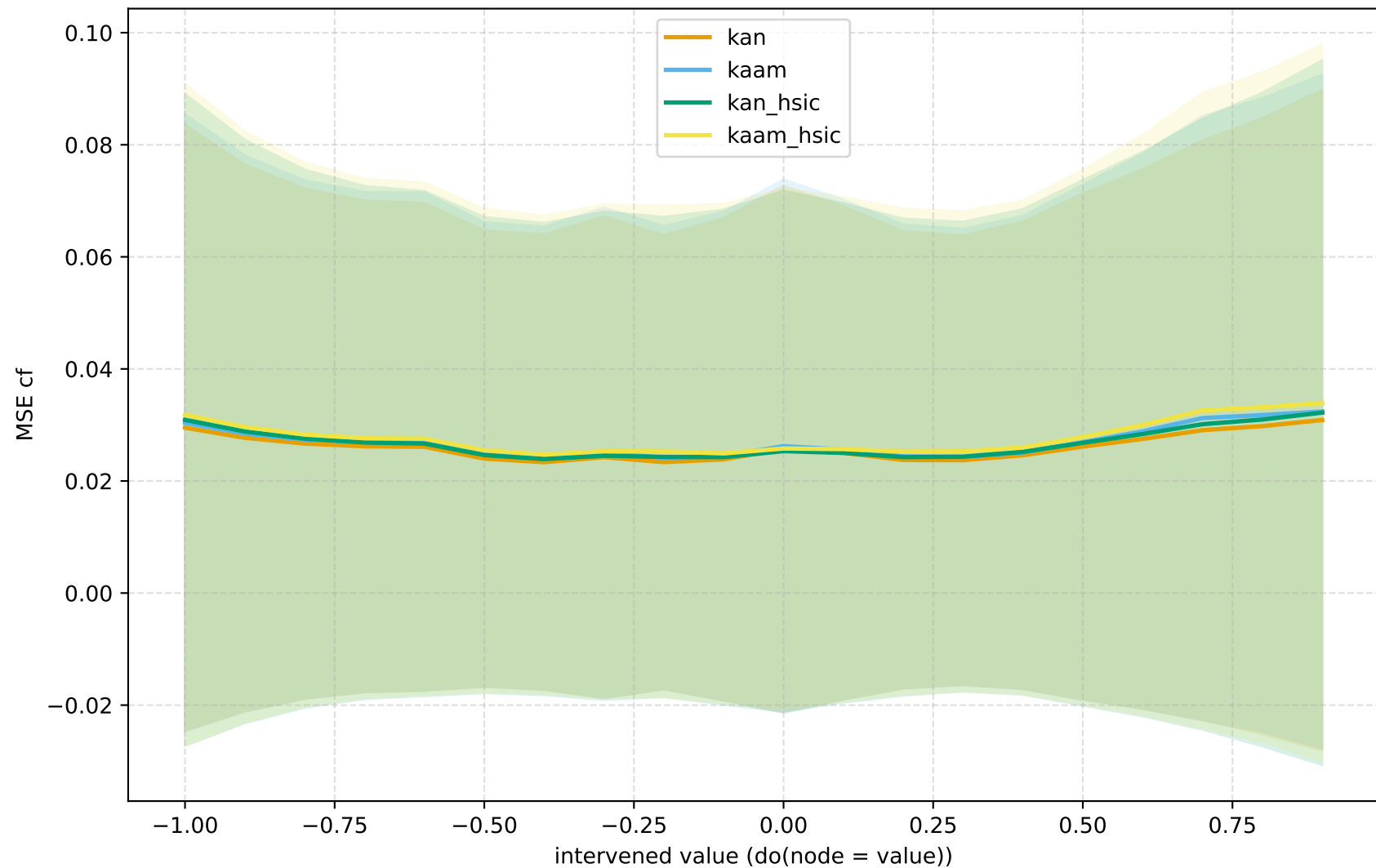
MSE cf vs intervention value (over 11 nodes)
