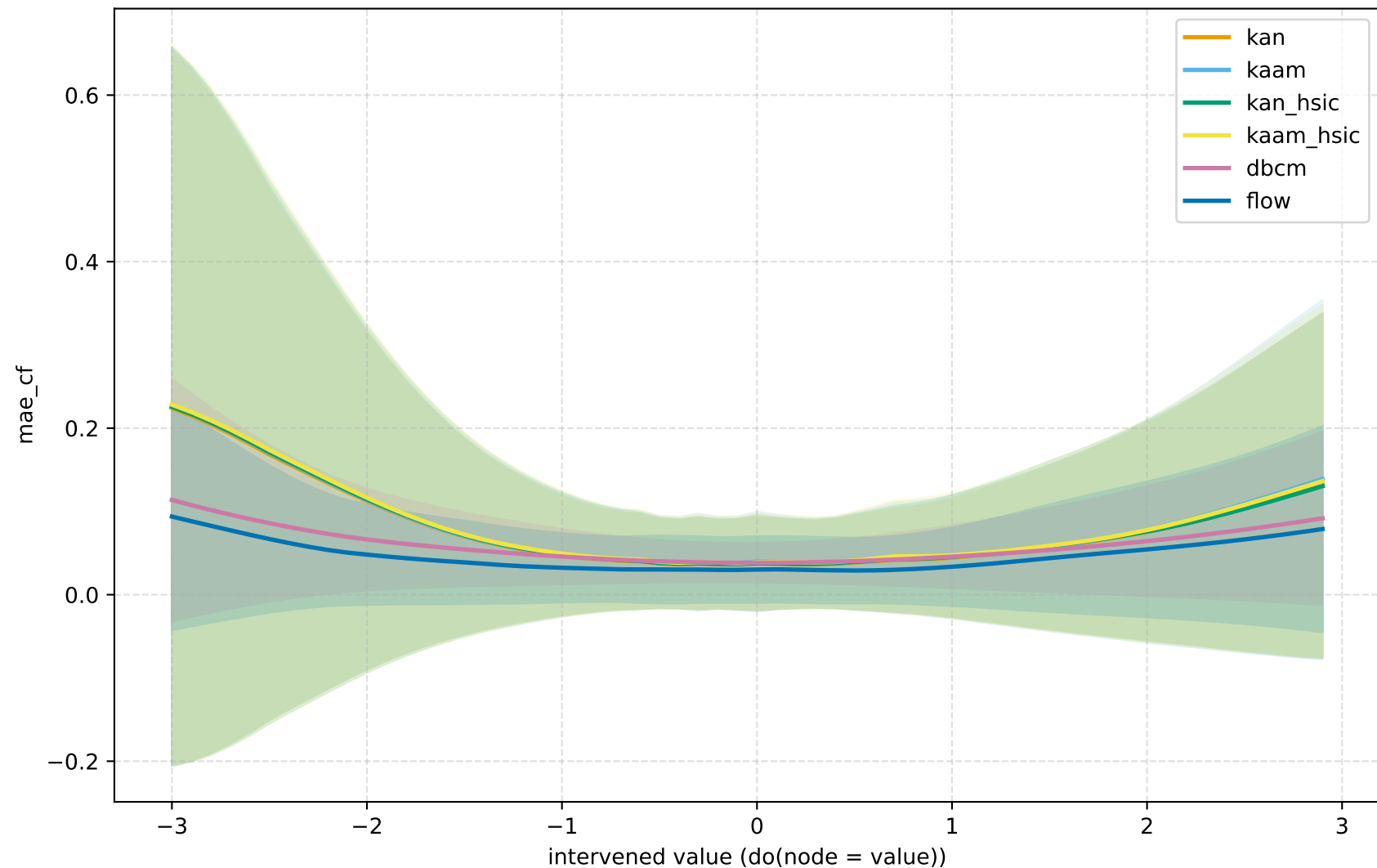
MAE (counterfactual) vs intervention value (media \pm std sobre los 11 nodos)
