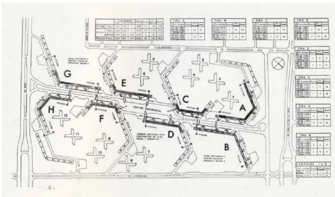
FIGURA 1. Lugano I y II. Planta de conjunto. Fuente: Comisión Municipal de la Vivienda. GCBA.
