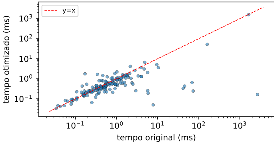
Tempo otimizado vs. original (Gemini 2.5 Flash Lite)
