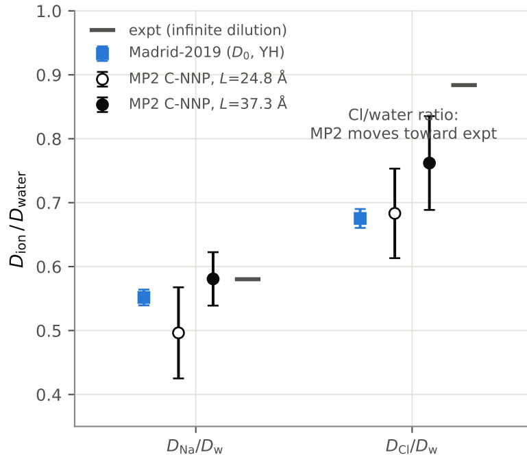
Ion/water diffusion ratio, 1 m
