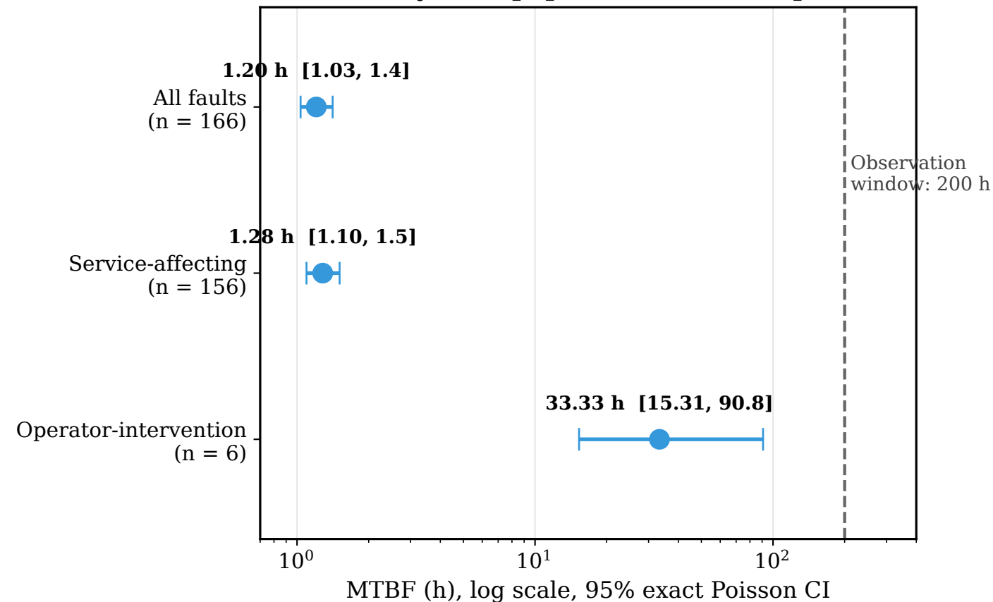
(d) MTBF by fault population (no extrapolation)
