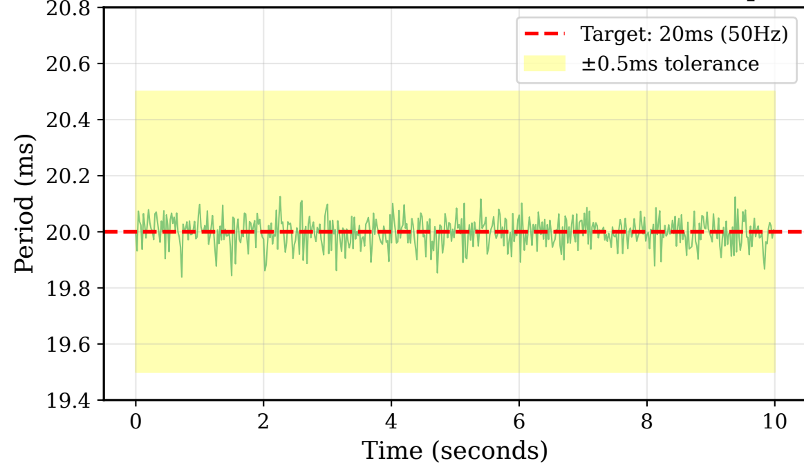
(d) WebSocket interval (max dev. 0.19 ms = 0.95% of period)
