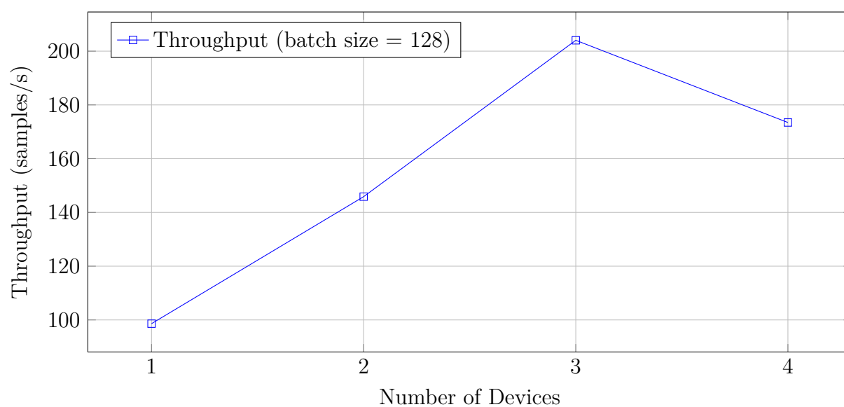
FIGURE 2.7 – Throughput en fonction du nombre de GPU (batch size = 128).
