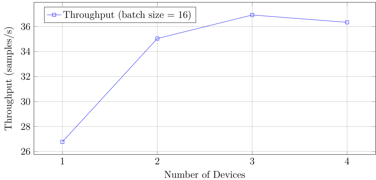
FIGURE 2.5 – Throughput en fonction du nombre de GPU (batch size = 16).
