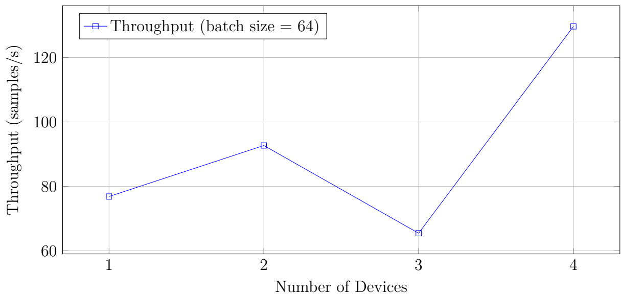
FIGURE 2.6 – Throughput en fonction du nombre de GPU (batch size = 64).
