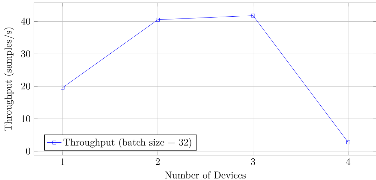
FIGURE 2.4 – Throughput en fonction du nombre de GPU.
