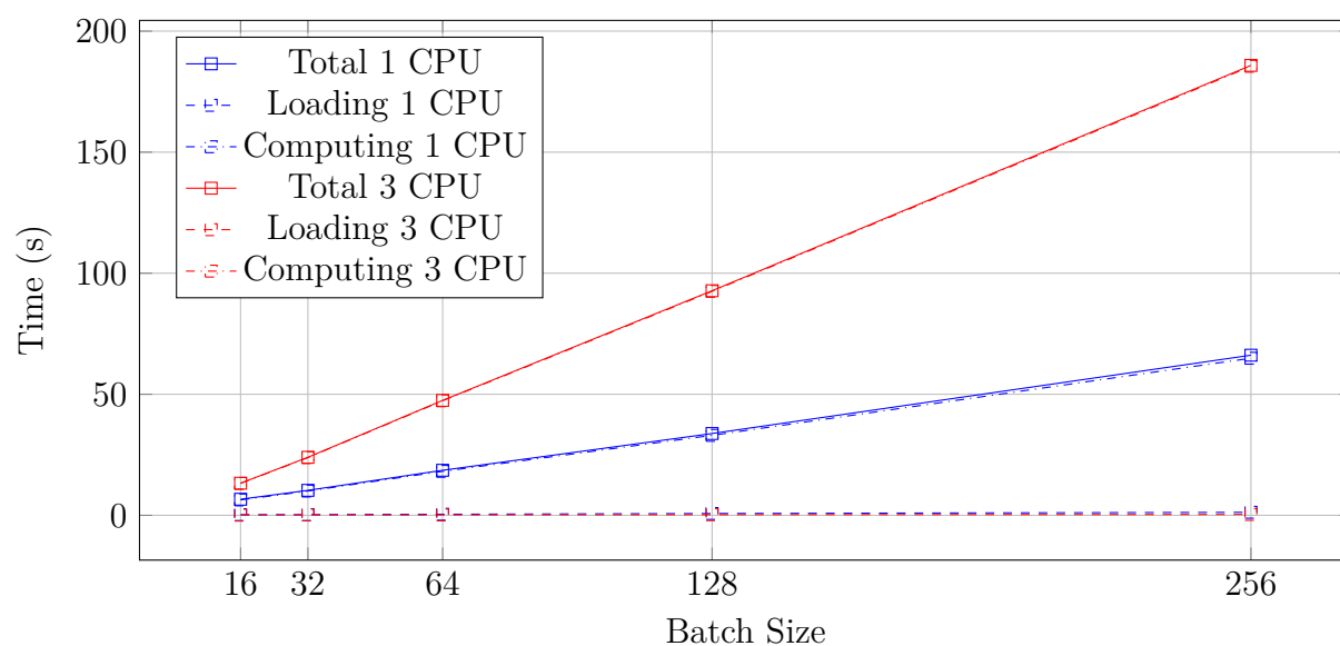
FIGURE 2.6 – Impact du batch size sur les temps de chargement et de calculs pour 1 et 3 CPU.
