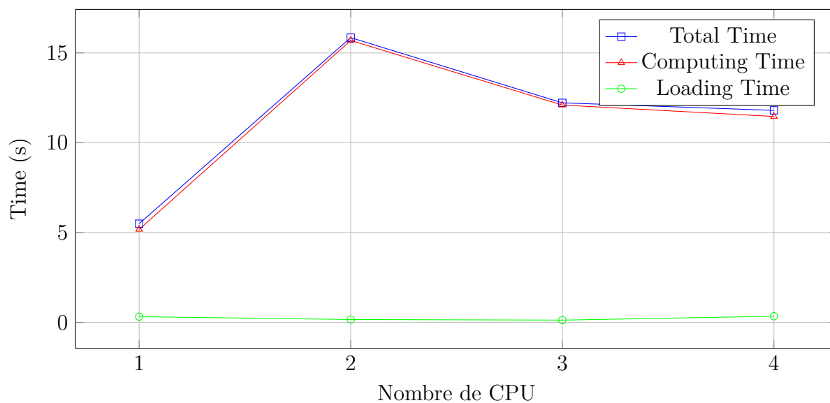
FIGURE 2.1 – Impact du nombre de CPU sur les temps d’entraînement.
