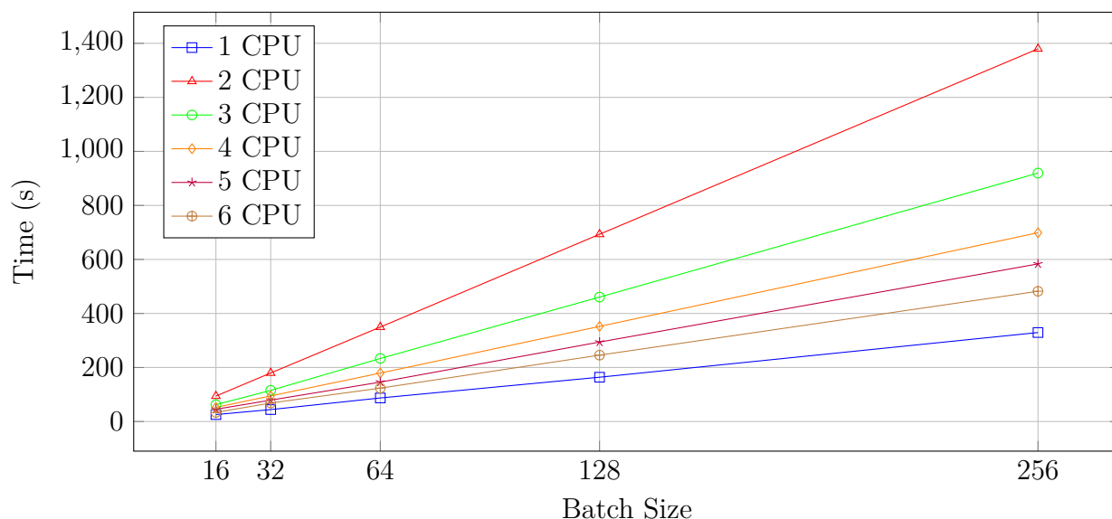
FIGURE 2.3 – Impact du batch size sur le temps total d'entraînement pour différents nombres de CPU.
