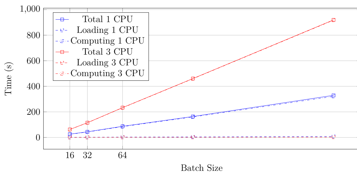
FIGURE 2.4 – Impact du batch size sur les temps de chargement et de calculs pour 1 et 3 CPU.
