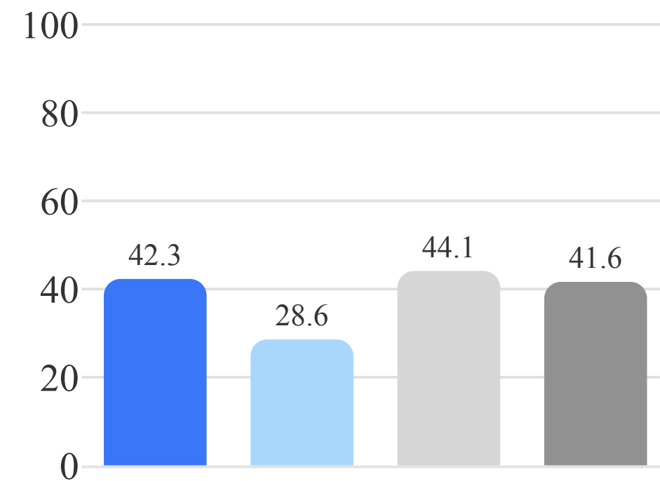
LiveCodeBench v6
