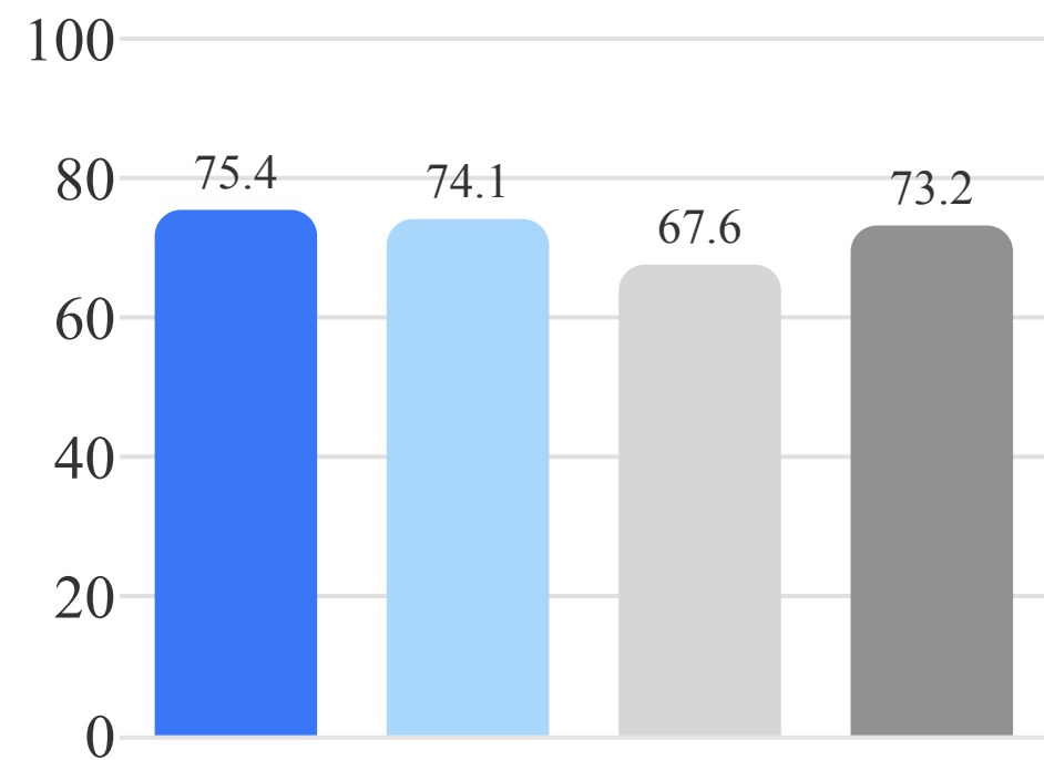
BFCL_Live
