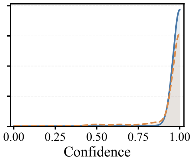
Gemma4-E2B
