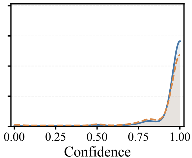
OLMo3-7B
