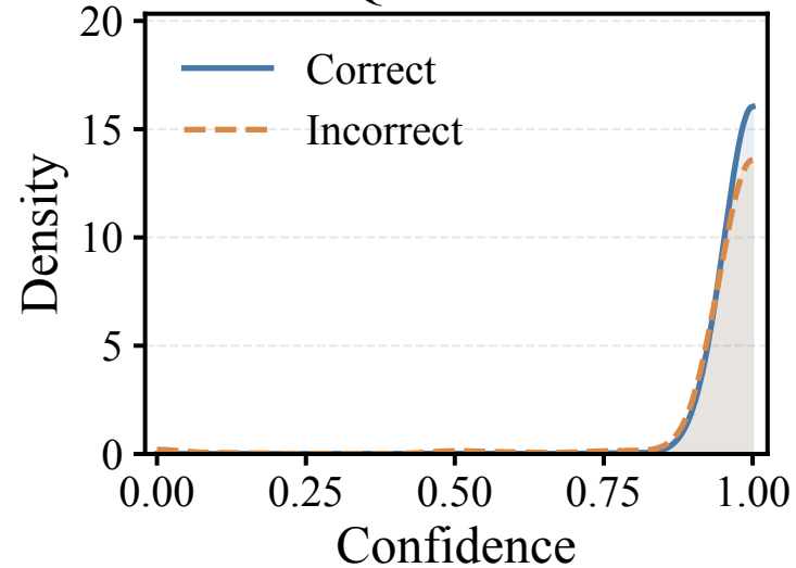
Qwen3-8B
