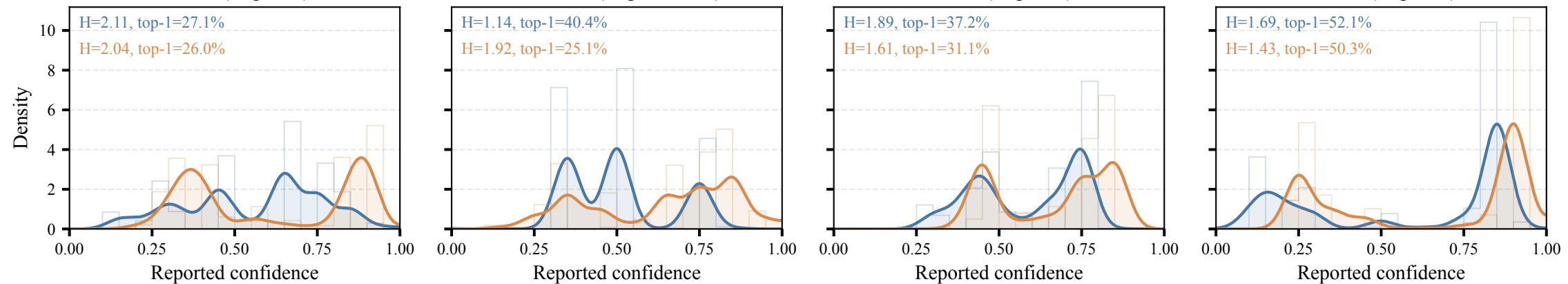
RLCR (step 160)
