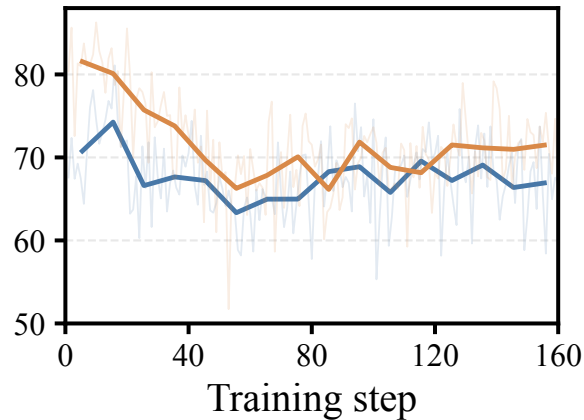
AUROC
