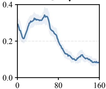
ECE ↓
