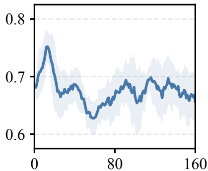
AUROC ↑
