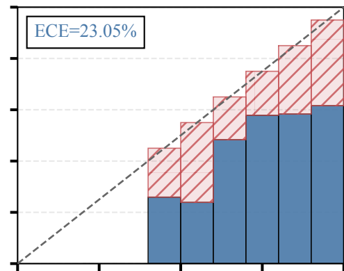
MinervaMath
