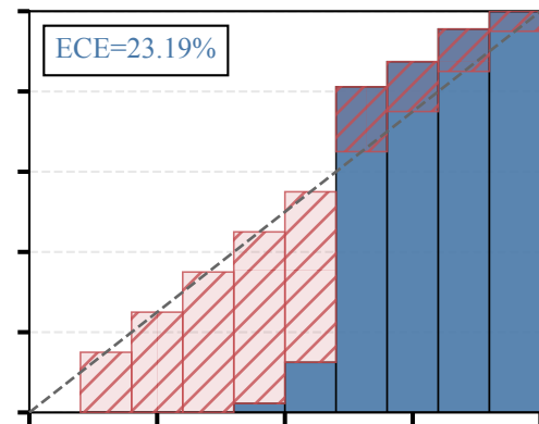
AIME 2026
