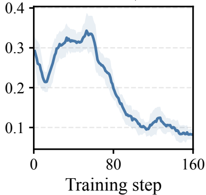
ECE ↓
