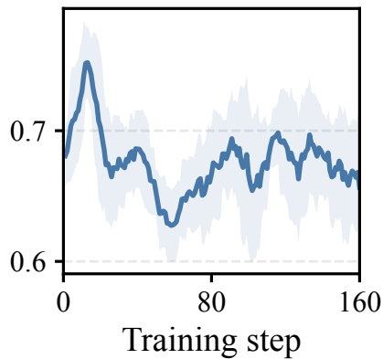
AUROC ↑
