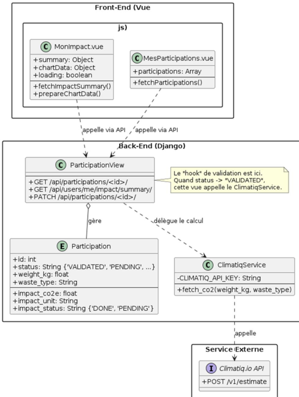
Diagramme de Classe - Feature "Calculateur d'Impact"
