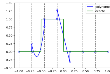
FIGURE 2 – Projection d'une fonction sur V_h avec peu de mailles. mauvais titre
