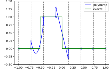
FIGURE 2 – Projection grossière d'une fonction sur V_h
