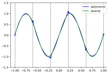
FIGURE 1 – projection d'une fonction sur V_h
