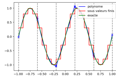
FIGURE 3 – Comparaison entre \underline{U} et \bar{U} .
