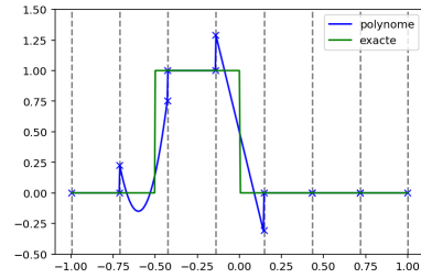
(11) FIGURE 2 – projection grossière d'une fonction sur V_h
