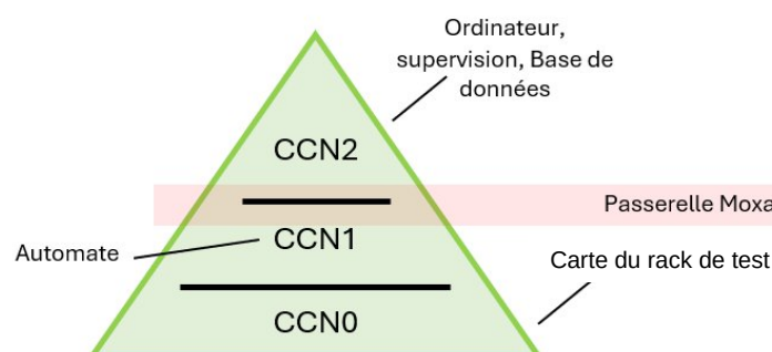
Figure 22 : Positionnement de la passerelle
