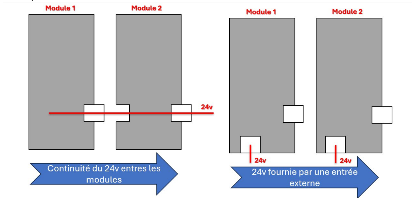
Figure 25 : Les deux types de connexion des modules
