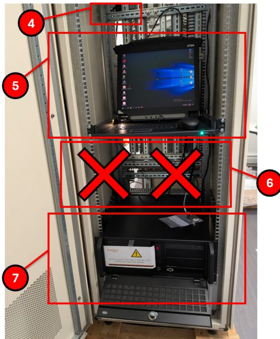
Figure 12 : Vue de l'avant
