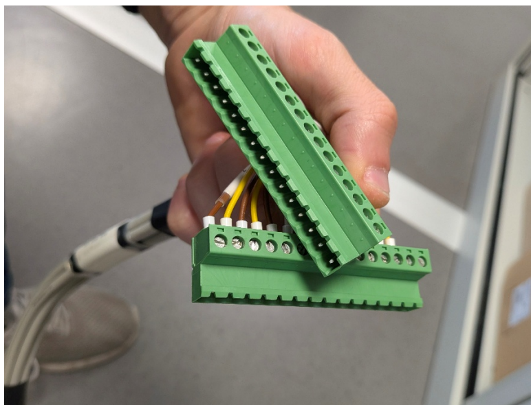
Figure 18 : connecteur Phoenix (Type femelle ici)
