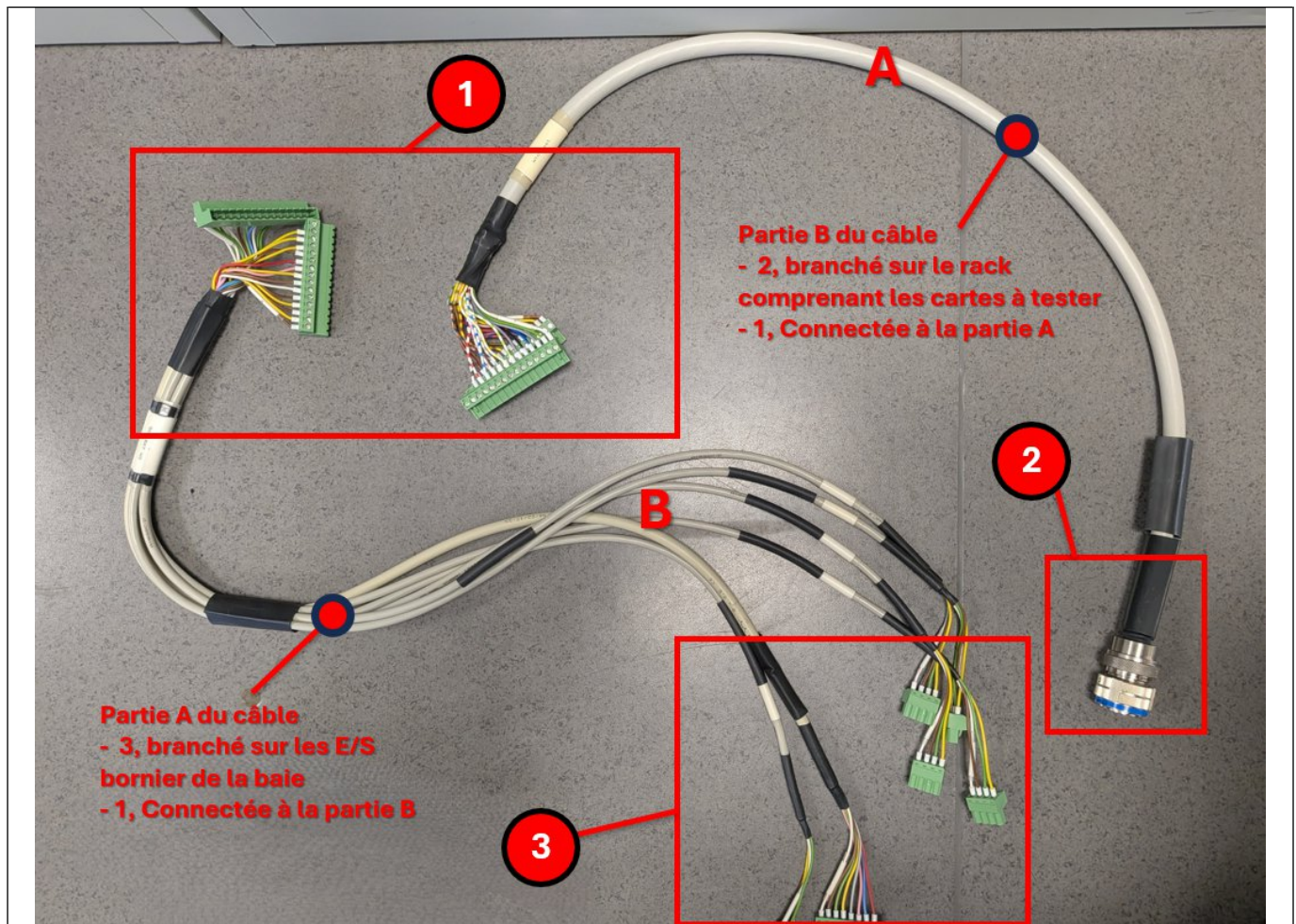
Figure 16 : Photo du câble de liaison Rack de test <=> Bornier
