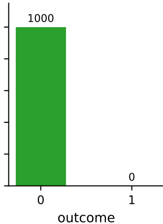
Y basis
