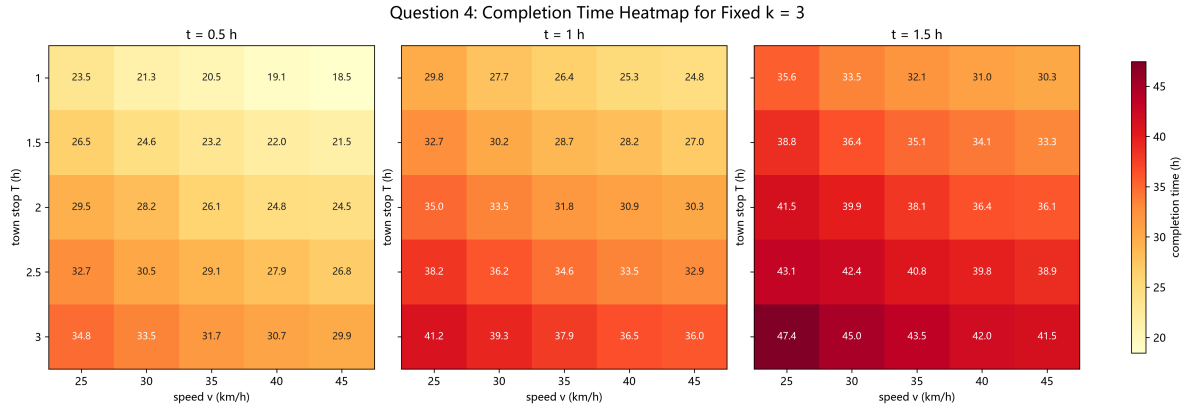
图 9: 第 (4) 问固定 k = 3 时的参数敏感性热力图。三个子图分别固定村停留时间 t , 横轴为车速 v , 纵轴为乡镇停留时间 T , 颜色和单元格数值表示该参数组合下重新优化得到的完成时间。
