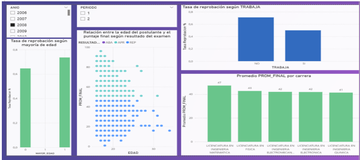
Figura 4-4: Dashboard de perfil general de los postulantes
