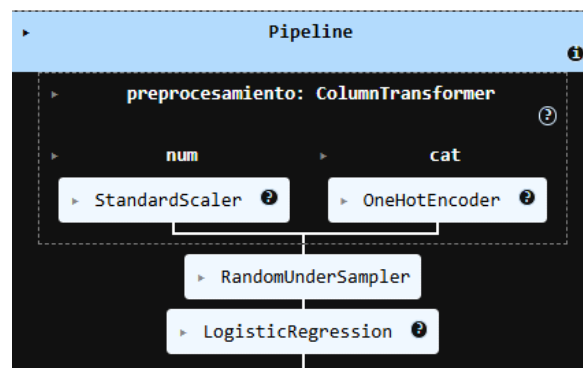
Figura 4-9: Pipeline creado para Regresión logística binaria
