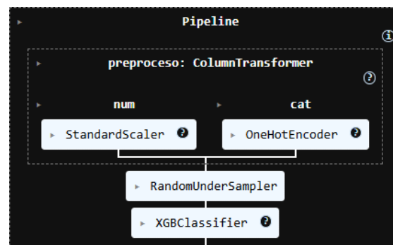
Figura 4-7: Pipeline creado para XGBoost Fuente: Elaboración propia, 2025
