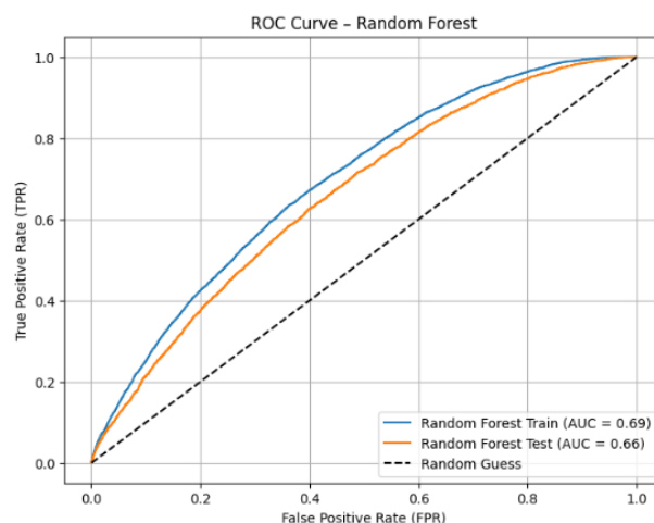
Figura 4-15: Grafica de curva de ROC del modelo Random Forest Fuente: Elaboración propia, 2025
