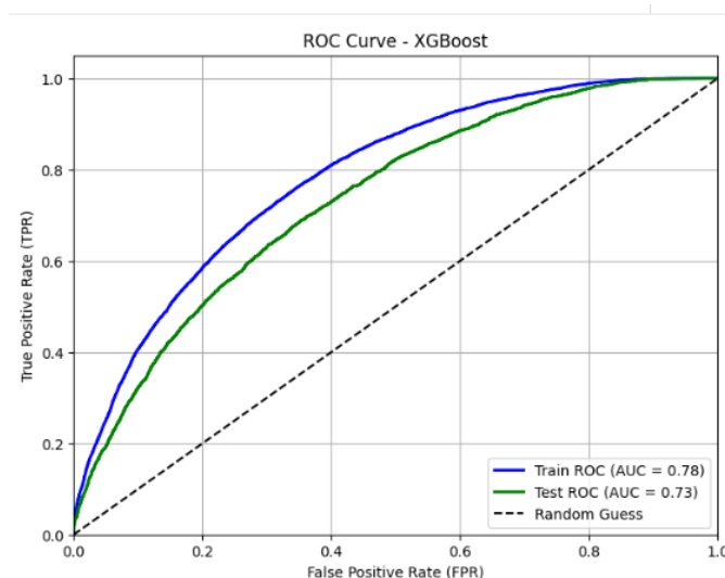
Figura 4-12: Grafica de ROC del modelo XGBoost
