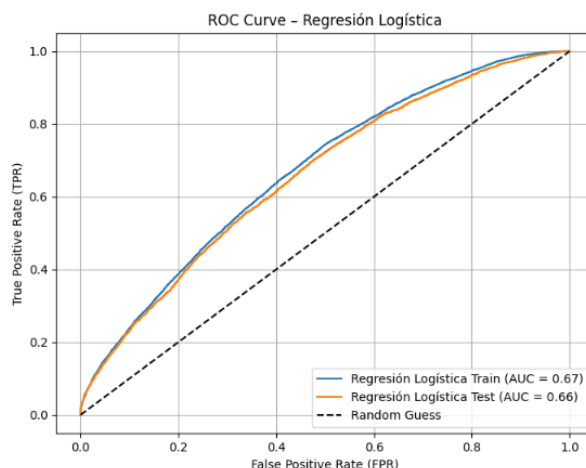
Figura 4-18: Grafica de curva de ROC del modelo de Regresión logística binaria Fuente: Elaboración propia, 2025
