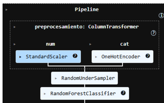
Figura 4-8: Pipeline creado para Random forest
