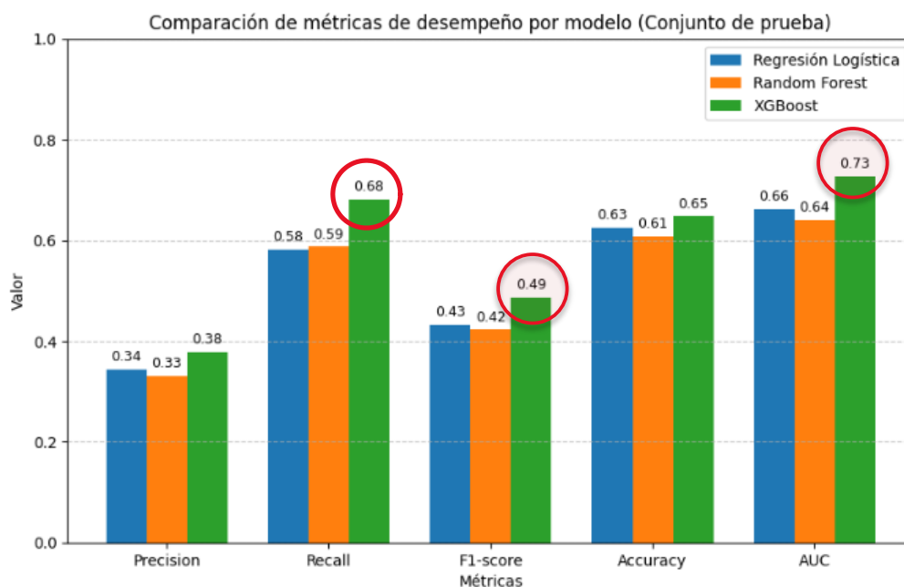
Figura 4-19: Comparación de métricas de desempeño de los modelos Fuente: Elaboración propia, 2025
