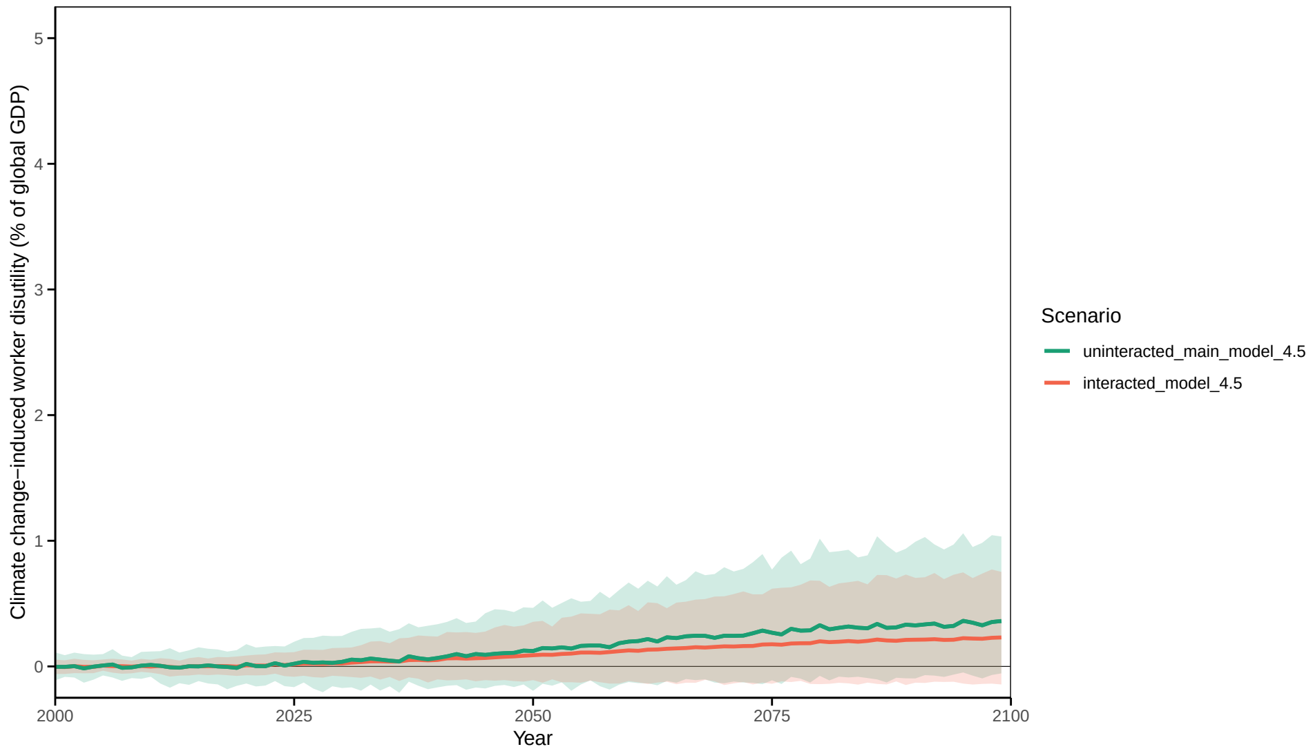
RCP4.5-SSP3-low
