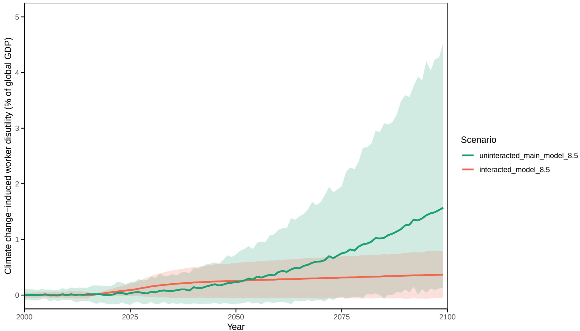
RCP8.5-SSP3-low
