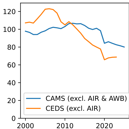
NMVOC
