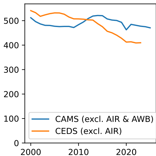
CO
