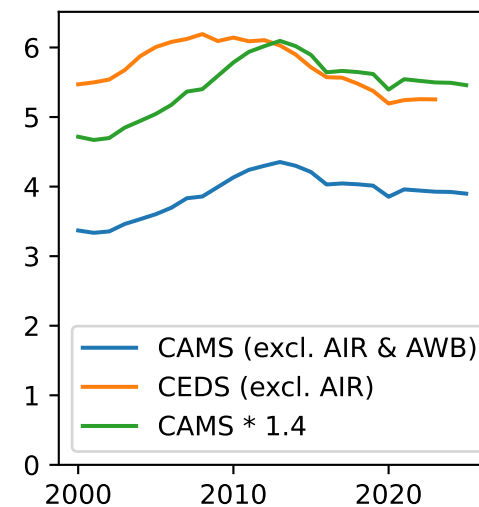
NO x
