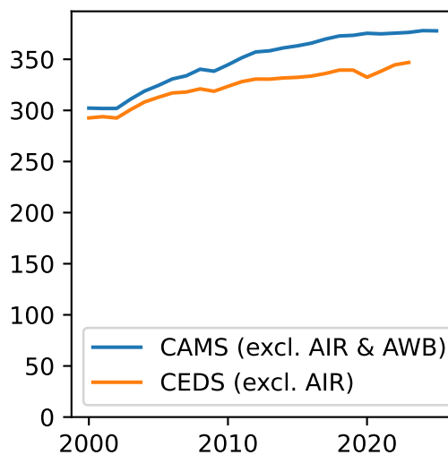
CH 4
