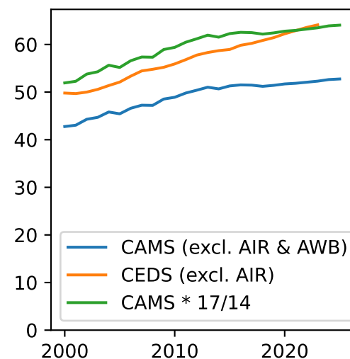
N 2 O
