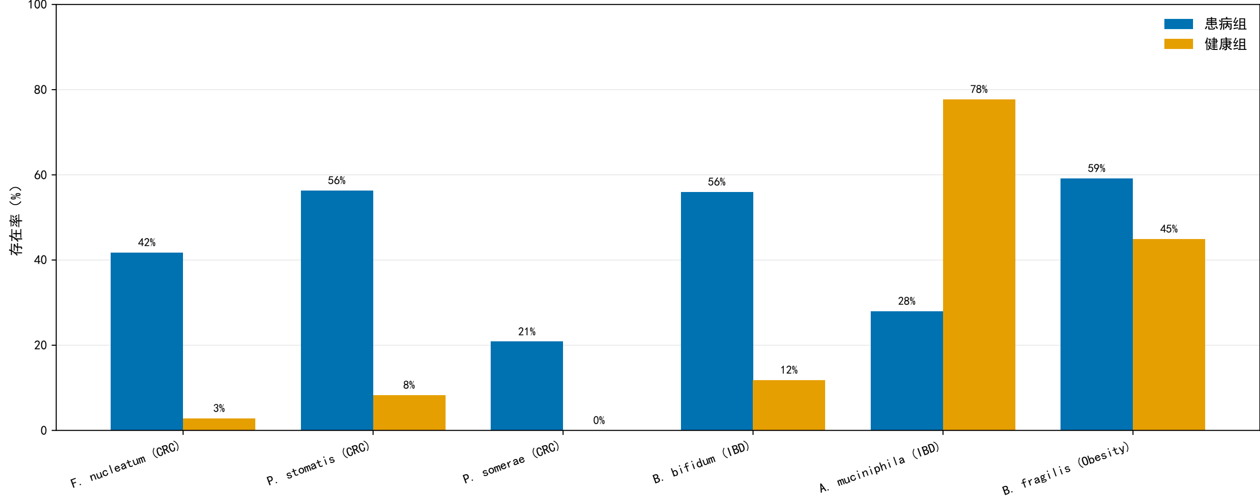
已知微生物标志物在患病/健康组的存在率对比
